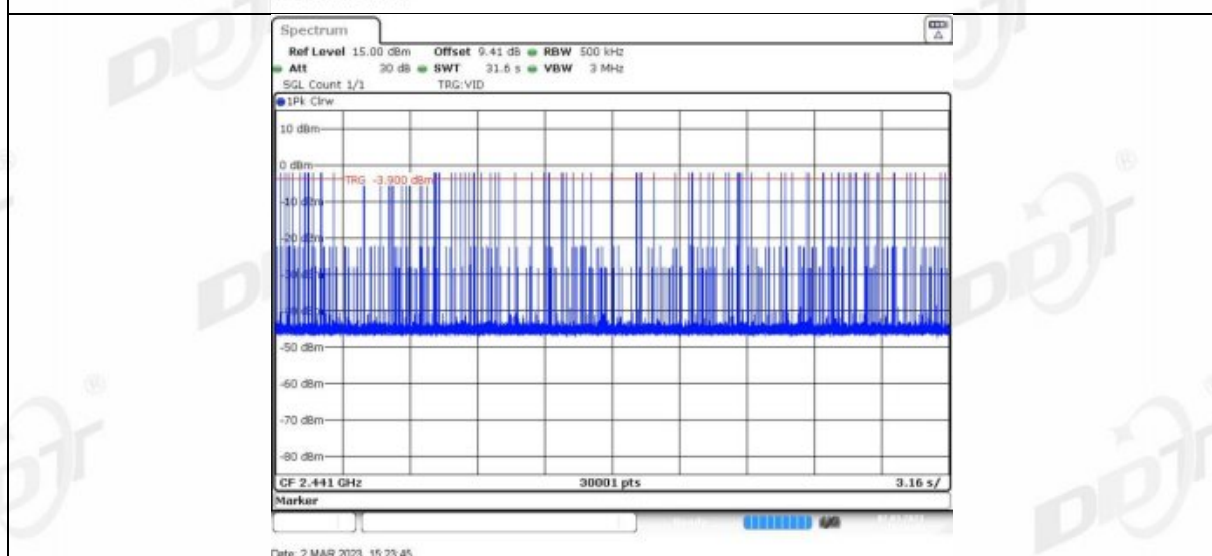
2DH1_Ant1_Hop
