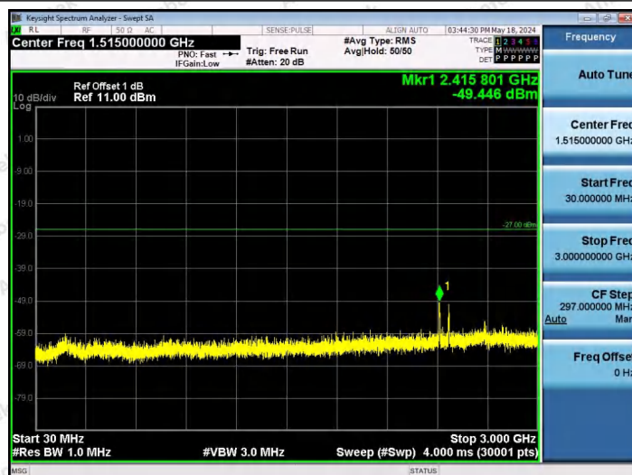
11AX40SISO-Ant1-6565-242Tone-RU62-30~3000-PASS
