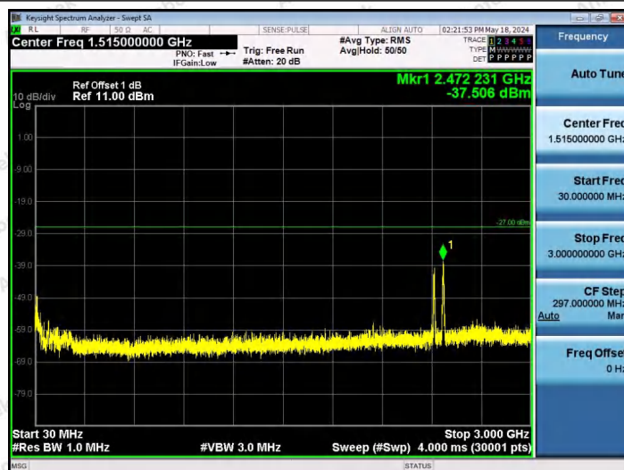
11AX40SISO-Ant1-6445-242Tone-RU62-30~3000-PASS
