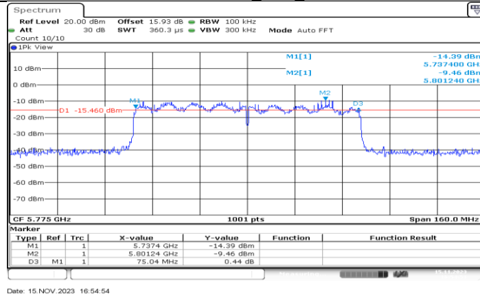
11AC80SISO_Ant1_5775
