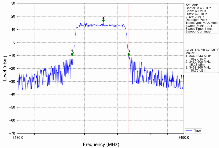
Band42a_20MHz_16QAM_LCH_3460MHz_RB_100_0_NTNV
