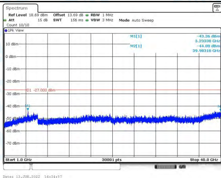
11AC40MIMO_Ant1_5270_1000~40000
