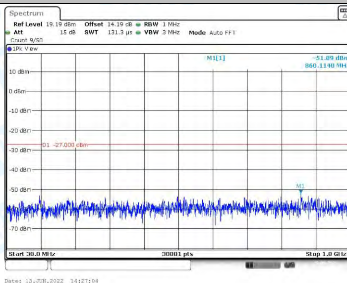
11AC20MIMO_Ant1_5700_30~1000
