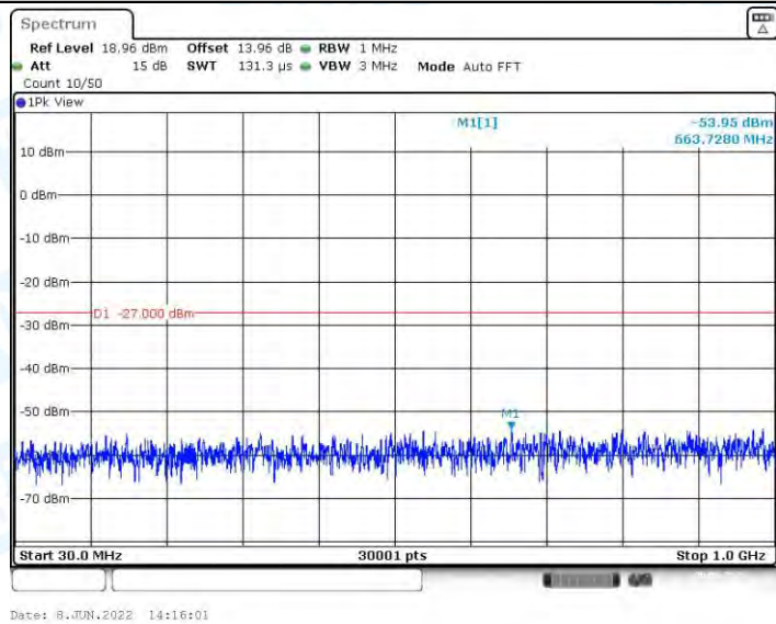
11AC20MIMO_Ant1_5825_30~1000
