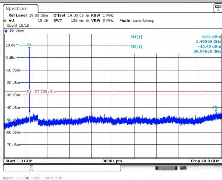
11AC40MIMO_Ant1_5510_1000~40000
