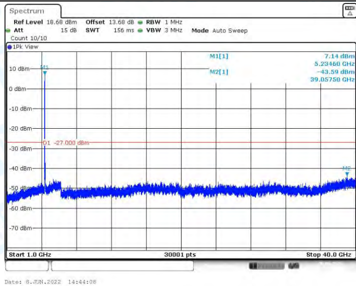
11AC40MIMO_Ant1_5230_1000~40000
