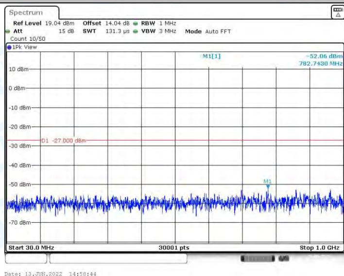
11AC40MIMO_Ant2_5550_30~1000
