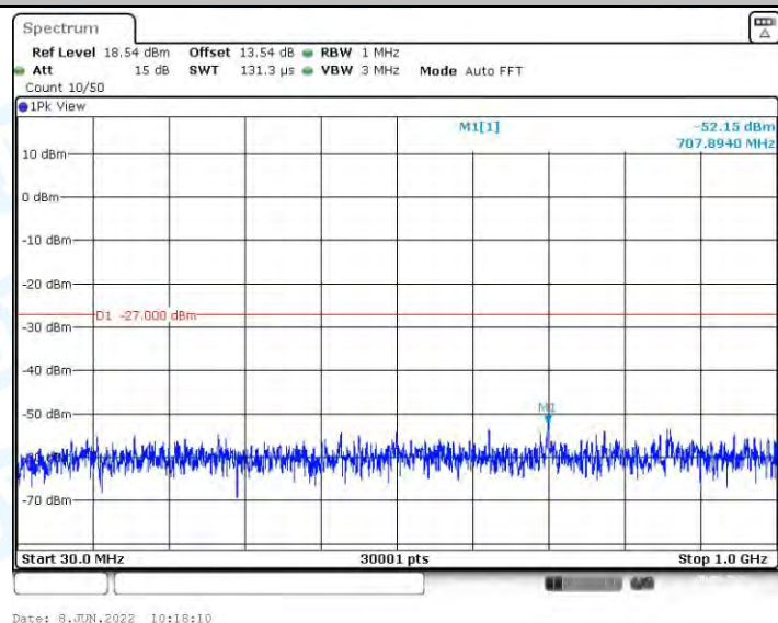
11N20MIMO_Ant1_5220_30~1000
