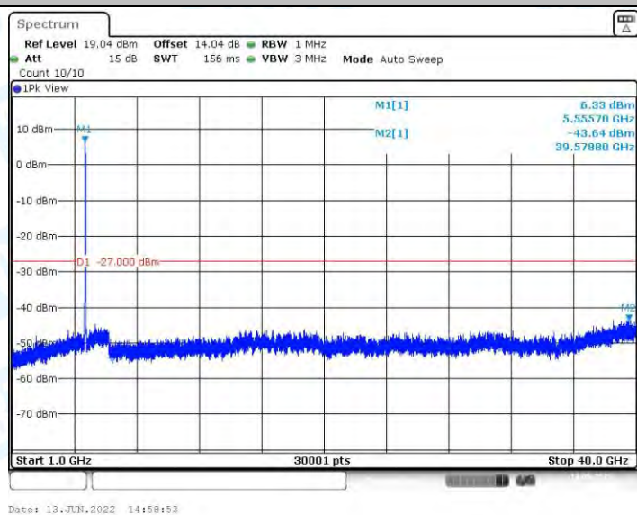
11AC40MIMO_Ant2_5550_1000~40000
