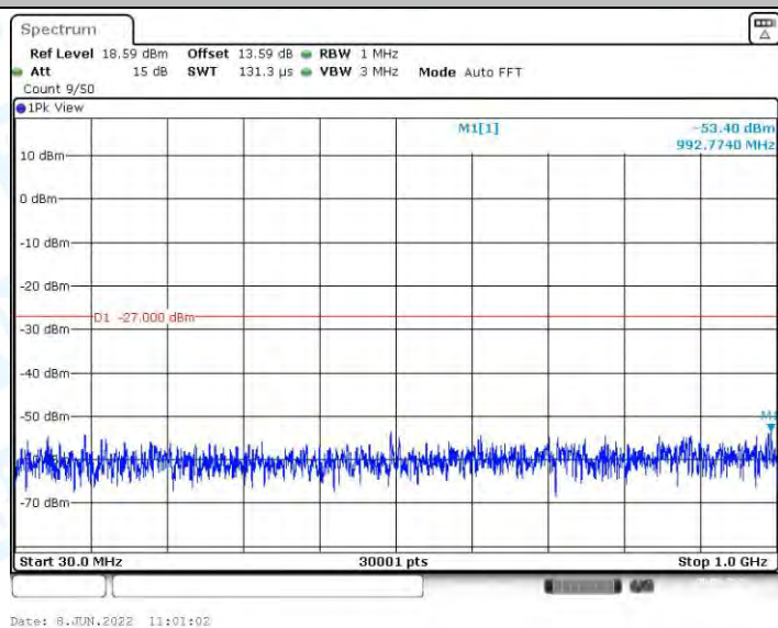
11N40MIMO_Ant2_5190_30~1000
