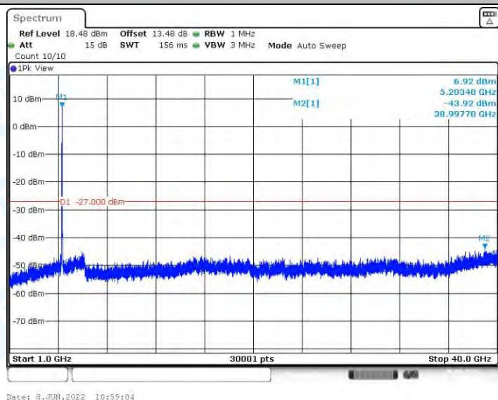
11N40MIMO_Ant1_5190_1000~40000
