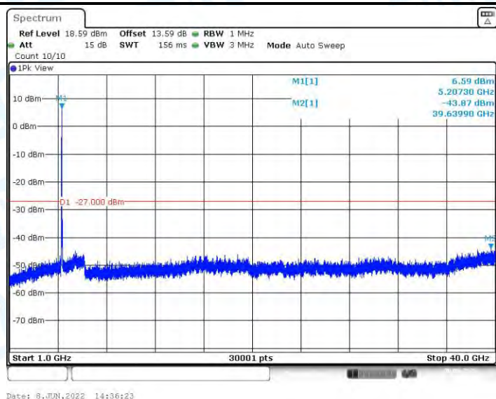
11AC40MIMO_Ant2_5190_1000~40000
