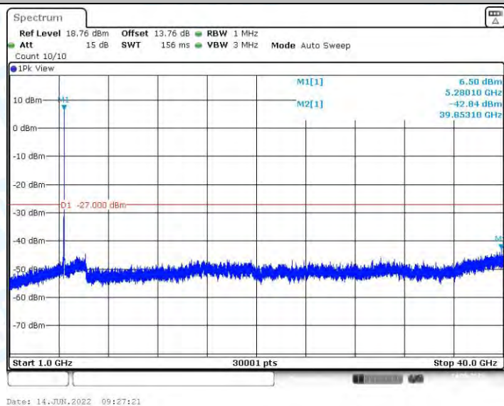
11AC40MIMO_Ant2_5270_1000~40000
