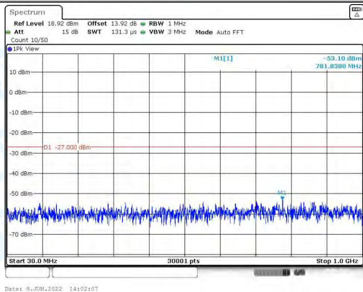
11AC20MIMO_Ant1_5785_30~1000
