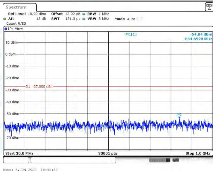
11N20MIMO_Ant1_5785_30~1000
