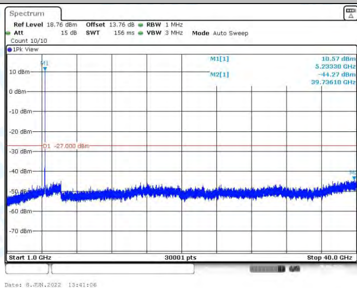
11AC20MIMO_Ant2_5240_1000~40000
