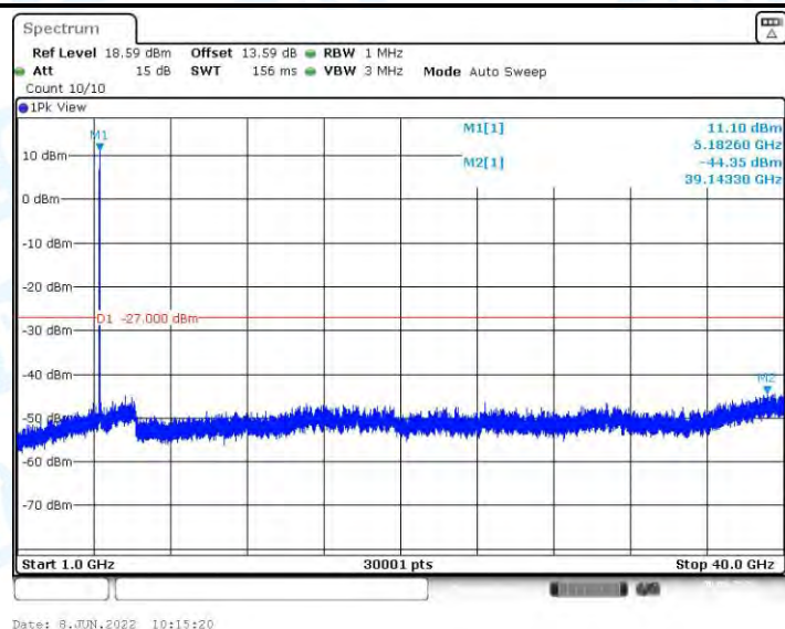
11N20MIMO_Ant2_5180_1000~40000
