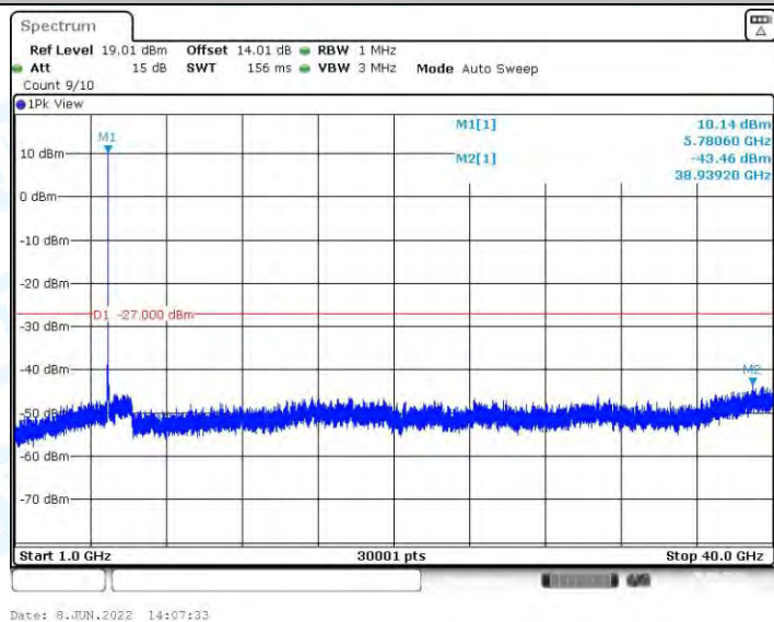
11AC20MIMO_Ant2_5785_1000~40000
