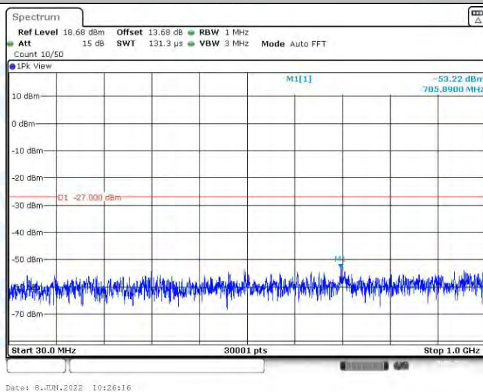
11N20MIMO_Ant1_5240_30~1000
