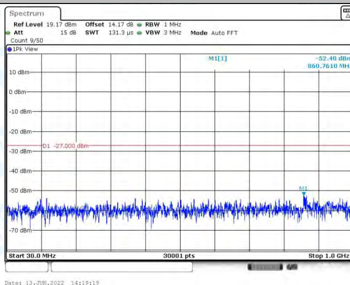
11AC20MIMO_Ant2_5500_30~1000
