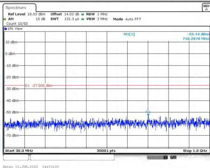
11AC40MIMO_Ant1_5510_30~1000
