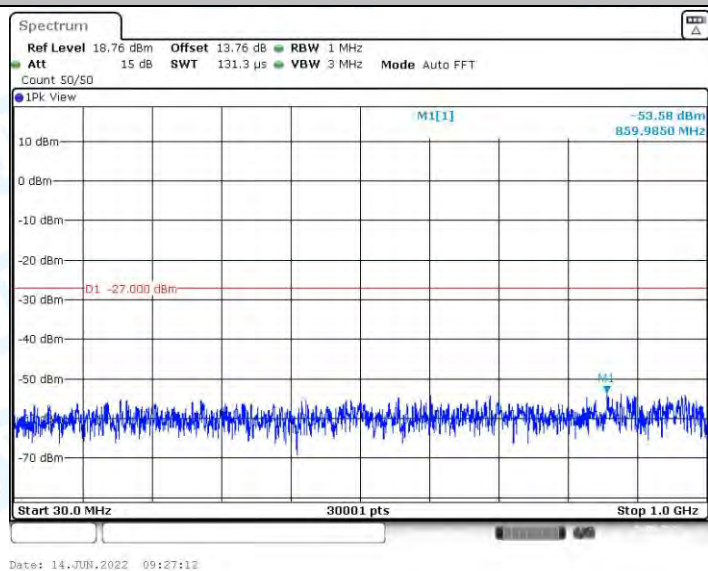
11AC40MIMO_Ant2_5270_30~1000
