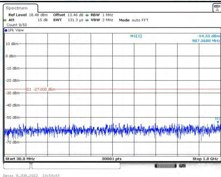
11N40MIMO_Ant1_5190_30~1000
