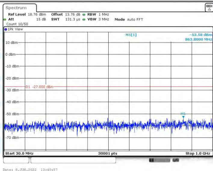
11AC20MIMO_Ant2_5240_30~1000
