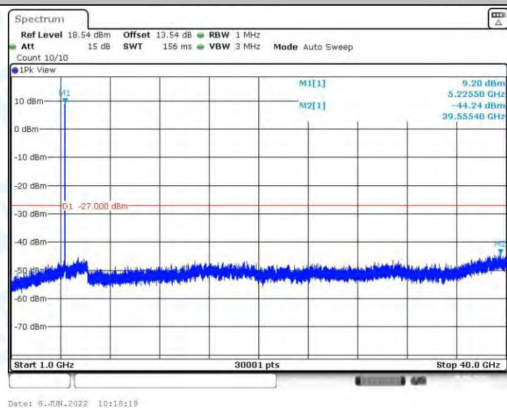
11N20MIMO_Ant1_5220_1000~40000
