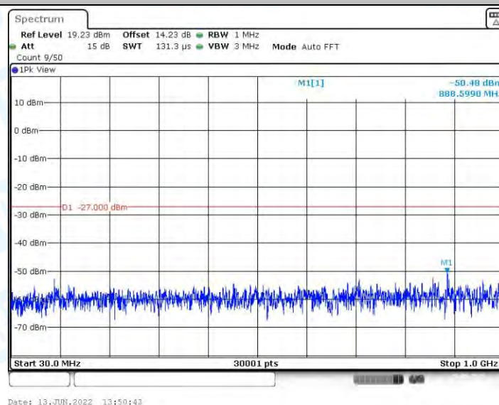
11N40MIMO_Ant2_5670_30~1000
