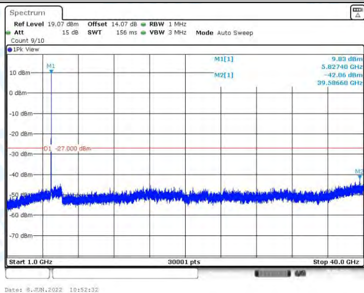
11N20MIMO_Ant2_5825_1000~40000
