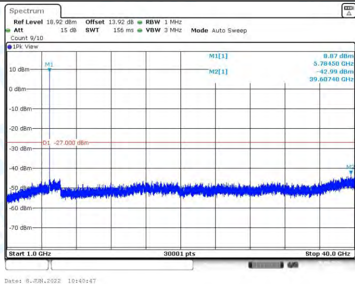
11N20MIMO_Ant1_5785_1000~40000
