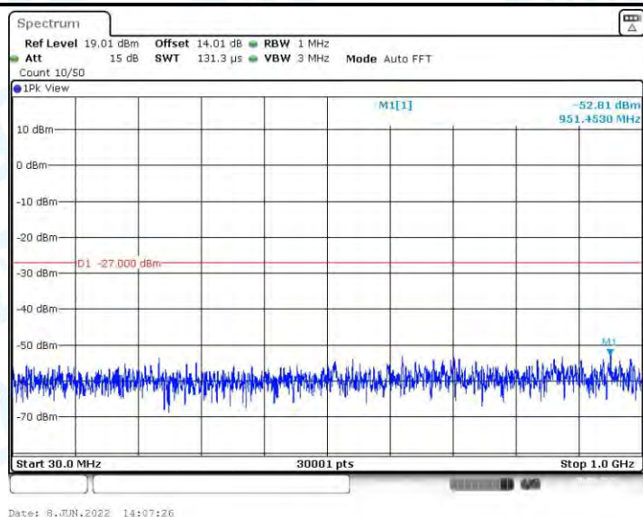
11AC20MIMO_Ant2_5785_30~1000
