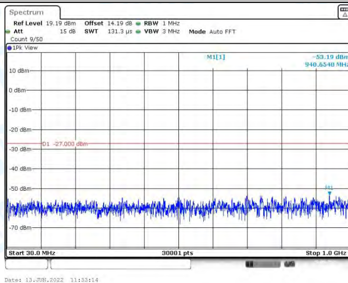
11N20MIMO_Ant1_5700_30~1000
