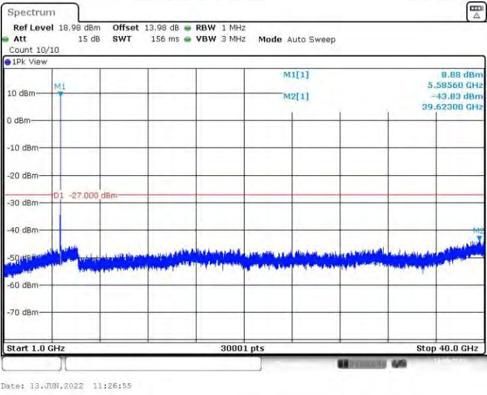
11N20MIMO_Ant1_5580_1000~40000
