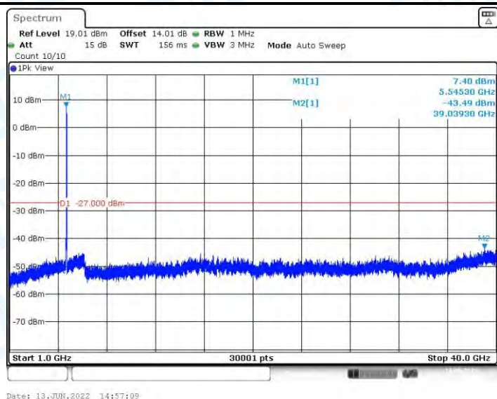
11AC40MIMO_Ant1_5550_1000~40000
