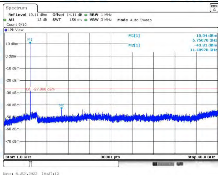
11N20MIMO_Ant2_5745_1000~40000
