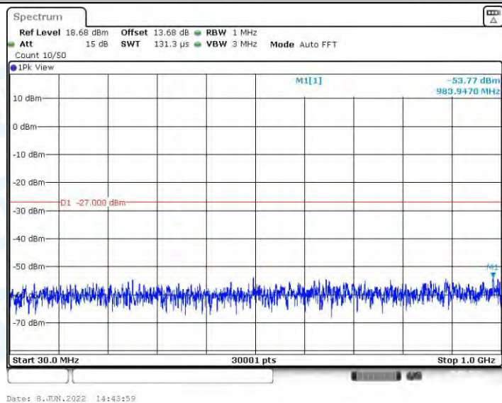
11AC40MIMO_Ant1_5230_30~1000
