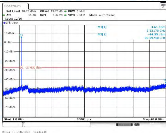
11AC40MIMO_Ant2_5310_1000~40000
