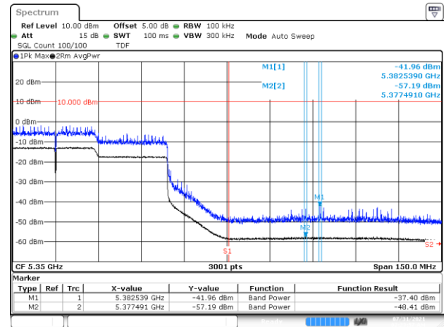
BE-R-HIGH, MIMO-A, 802.11ax160-HE0, Ch50
