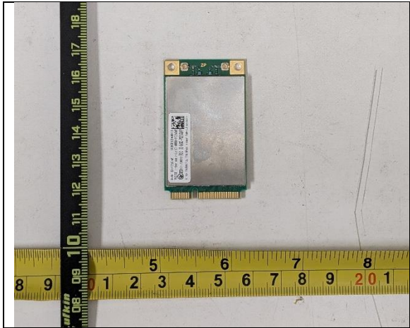
EUT-External-Front
