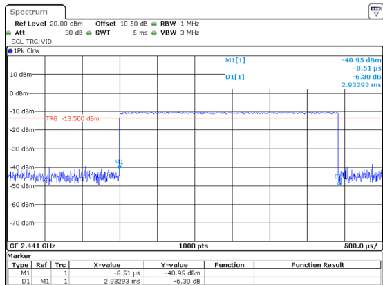
DH5_Hopping 2.933ms
