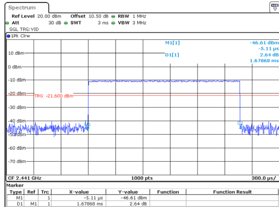
DH3_Hopping 1.679ms
