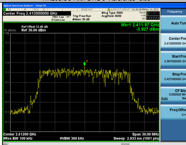
11N20SISO-Ant1-2412-30~1000--3.93
