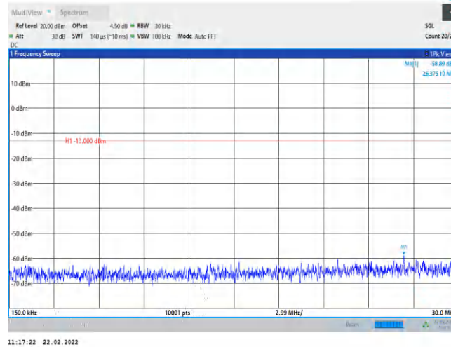
GSM850-128-3-0.15~30MHz
