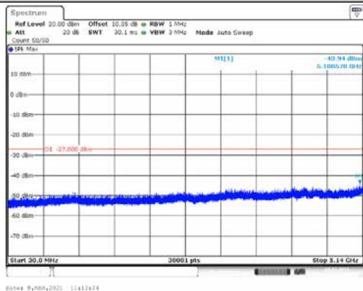
11A_Ant2_5260_30~5140
