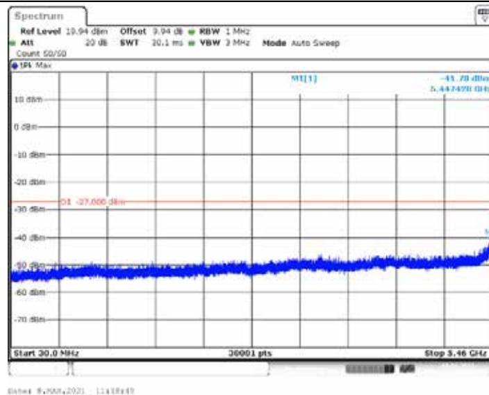
11N20SISO_Ant2_5500_30-5460
