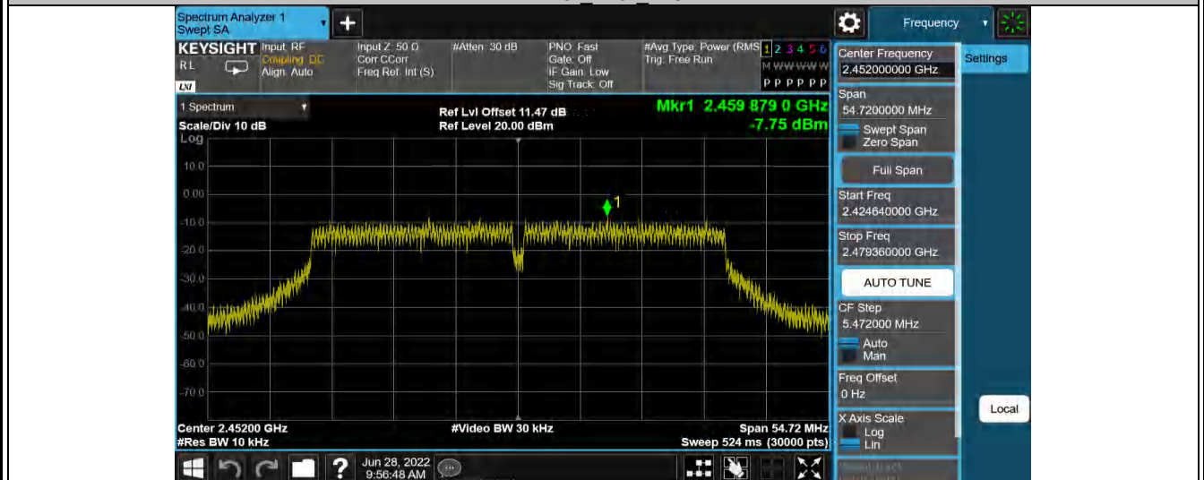
11N40- Ant1 2452
