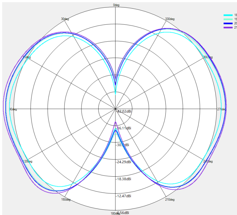
DCS/PCS/WCDMA B1/B2/B4/LTE B1/B2/B3/B4/B66 Theta=0deg
