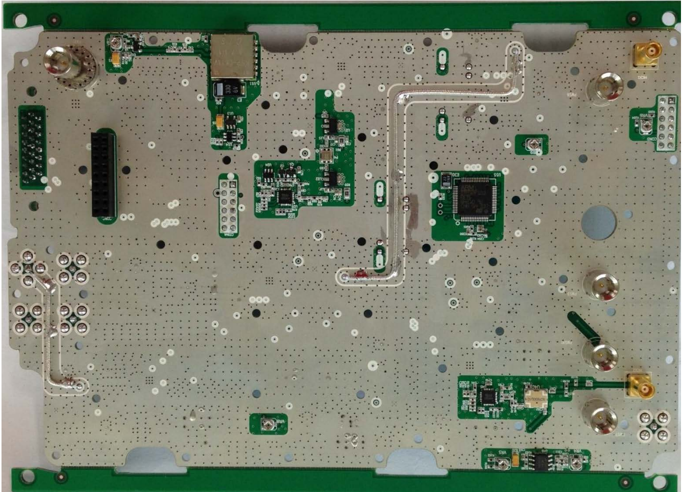
UDC PBA Bottom
