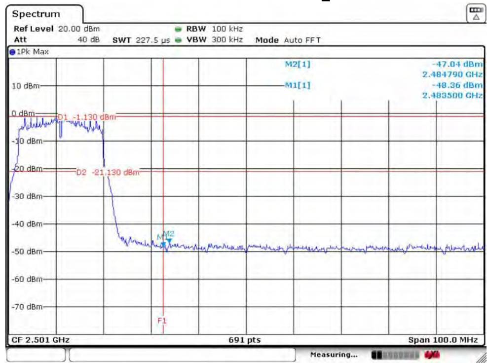
IEEE 802.11n HT20 2462MHz_ANT 2
