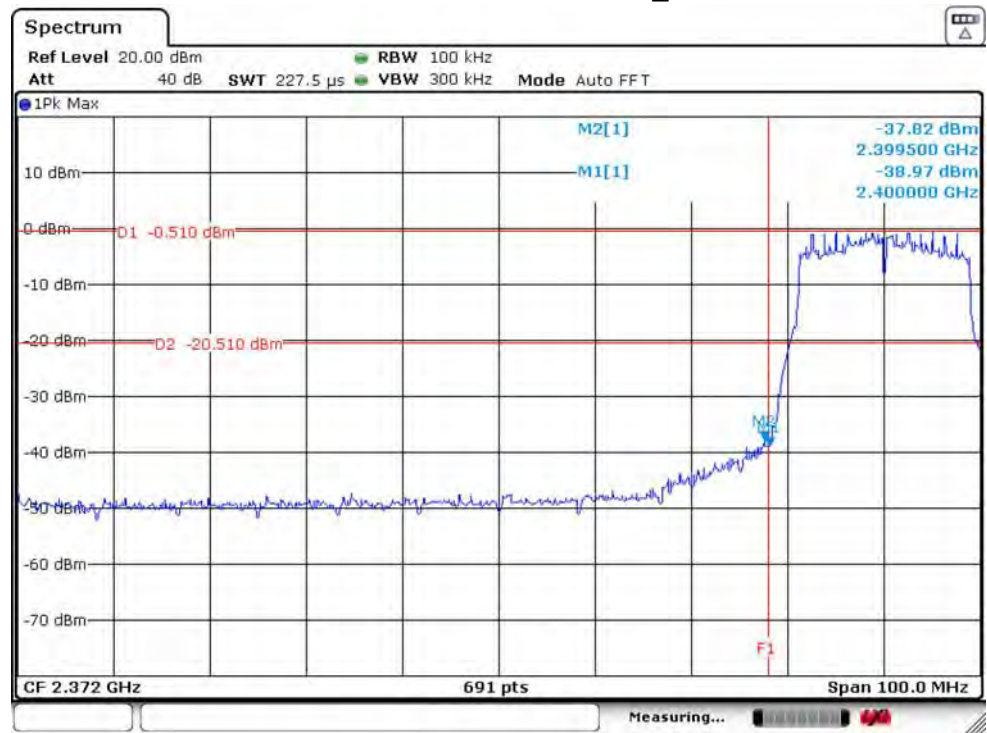
IEEE 802.11n HT20 2412MHz_ANT 2
