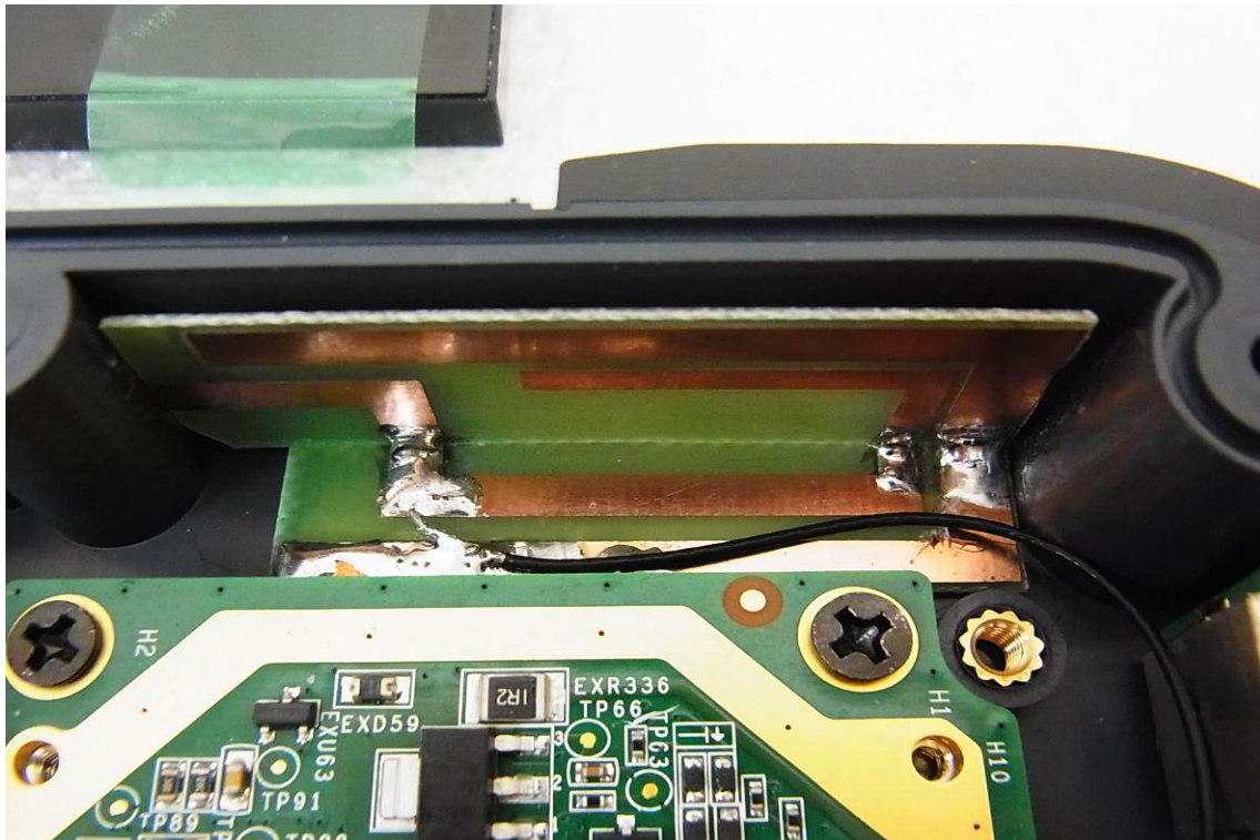
EUT 10 WWAN antenna2
