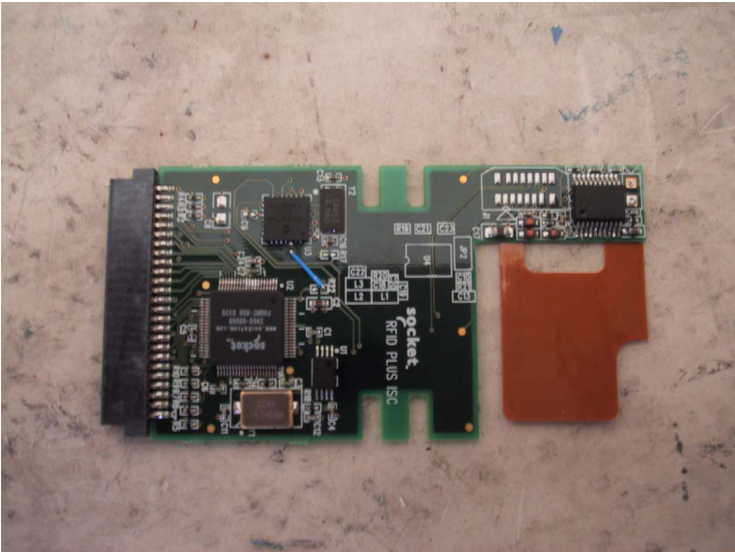
EUT PCB – Top Side
