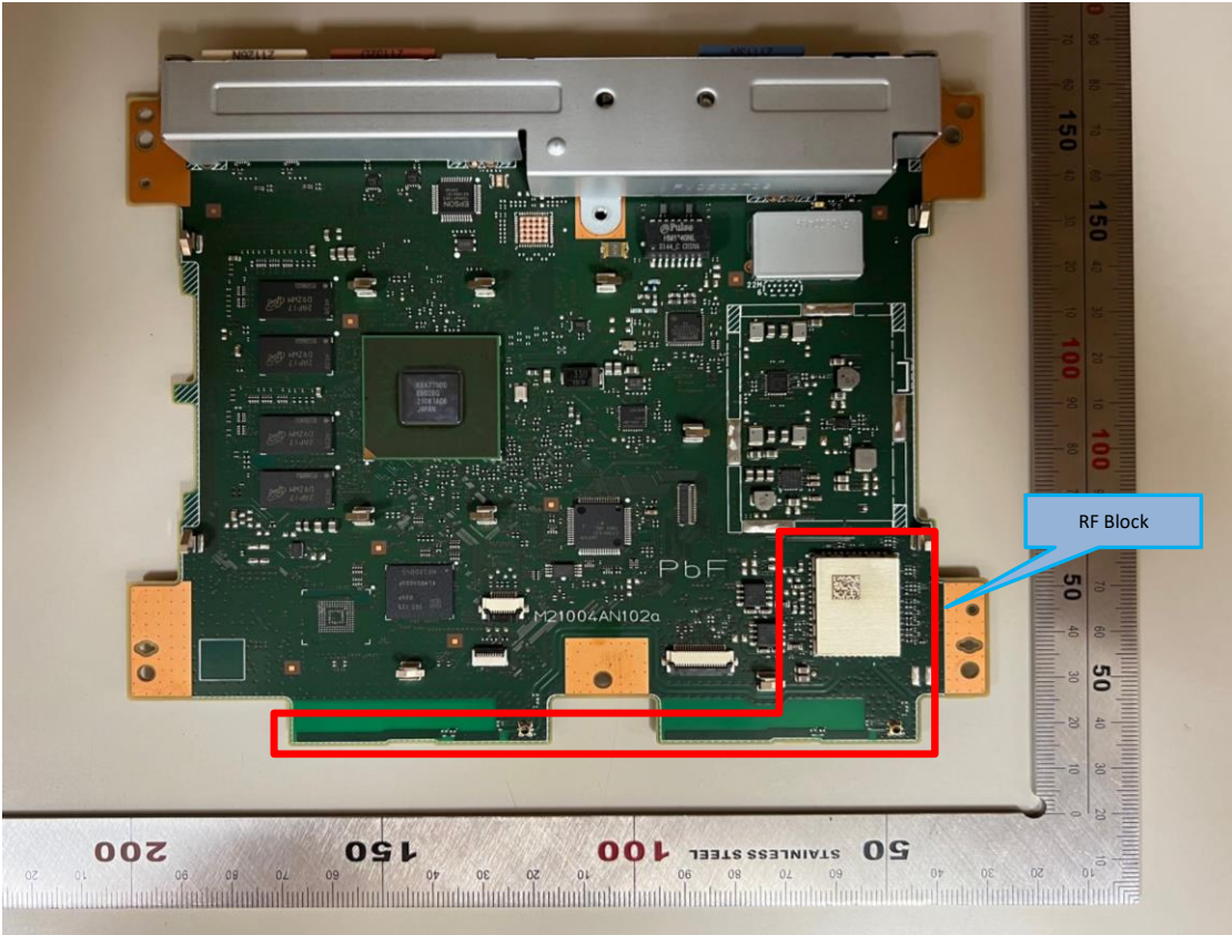
<BT/WLAN Block Zoom Up> 【Figure 2】
