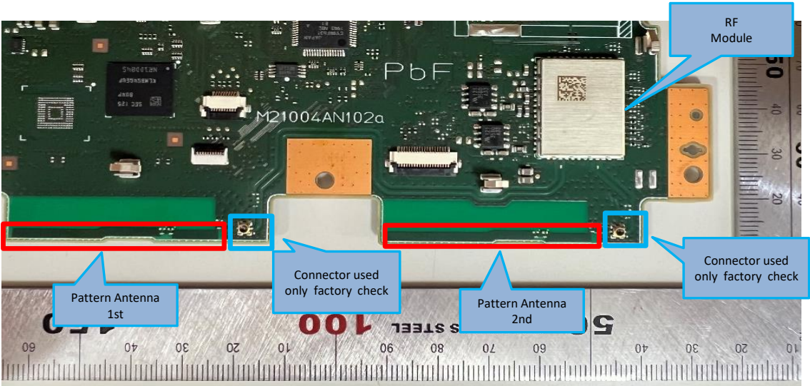
<BT/WLAN Block Zoom Up> 【Figure 2】
