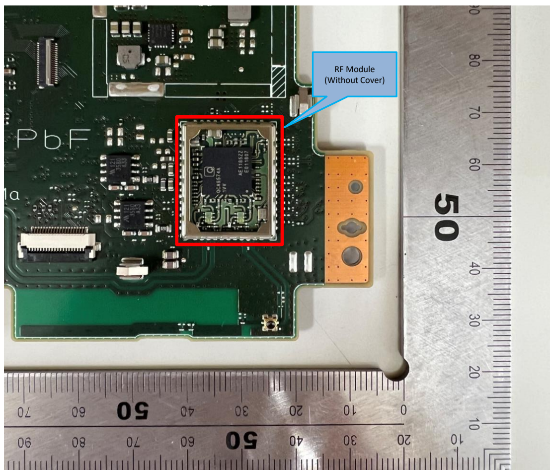
NAVI PCB Back Side 【Figure 4】
