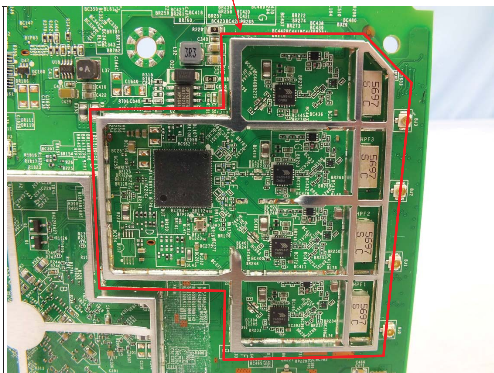
5G U-NII-3 Band Module (Brand: Cascade)
