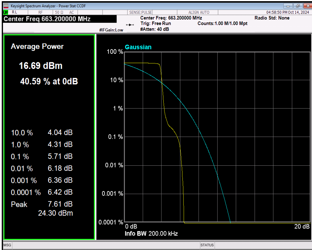
Band71 BPSK Channel=133124 nTones=1@0 Spacing=15kHz
