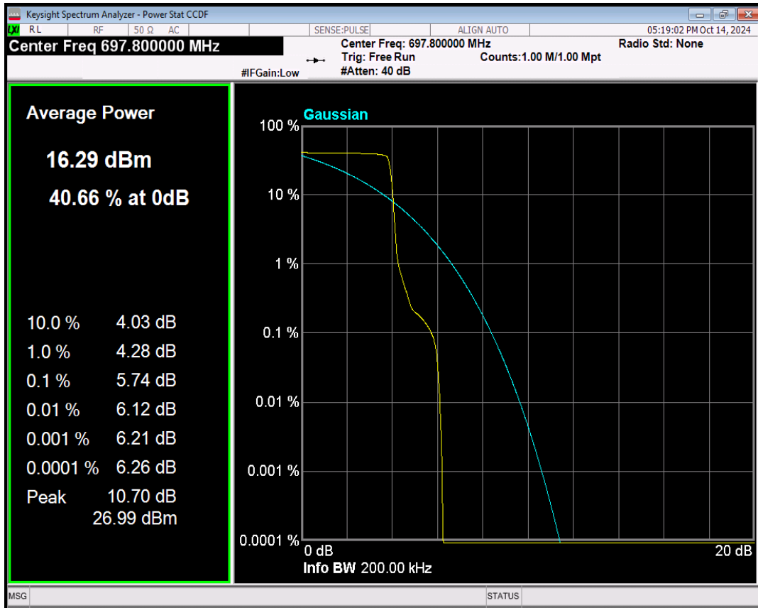
Band71 BPSK Channel=133470 nTones=1@0 Spacing=15kHz
