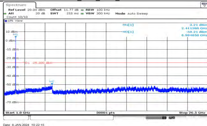
11B_Ant2_2412_1000~26500
