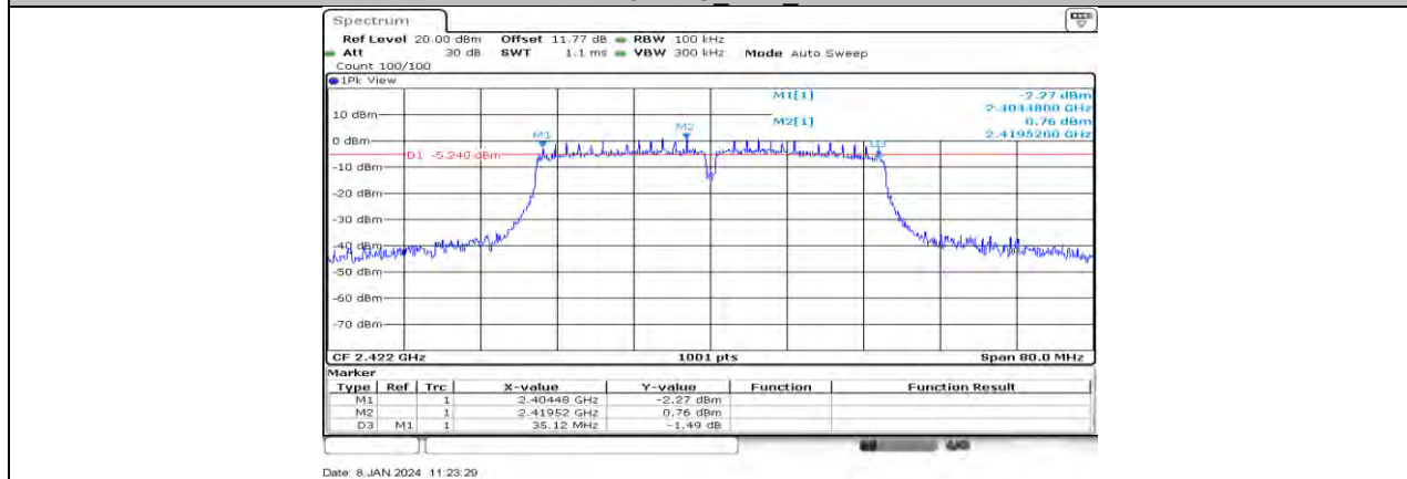
11N40MIMO_Ant2_2422
