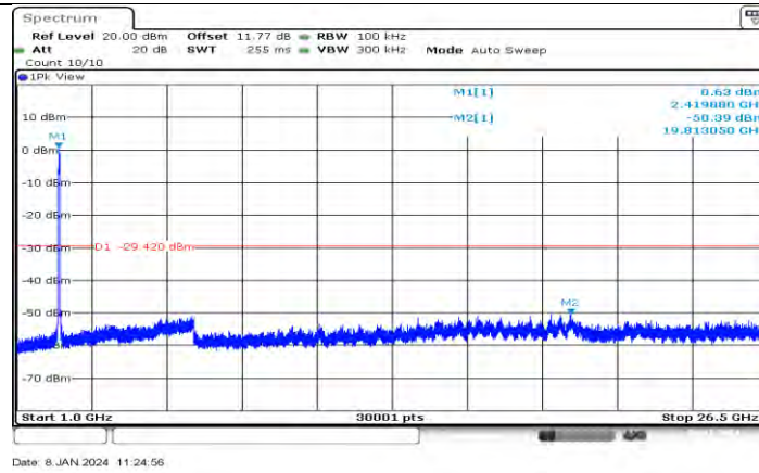
11N40MIMO_Ant2_2422_1000~26500
