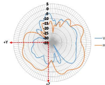
YZ-plane 6125 MHz
