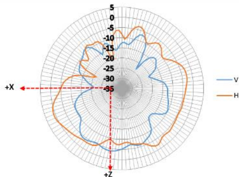
XZ-plane 6225 MHz
