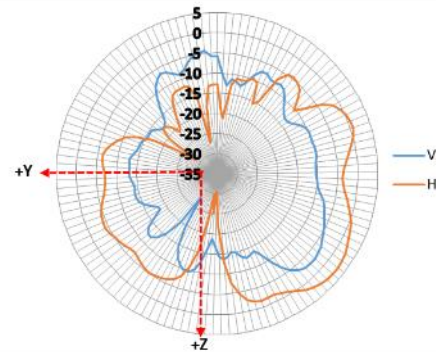
YZ-plane 6000 MHz
