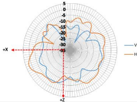
XZ-plane 6425 MHz
