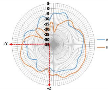
YZ-plane 6225 MHz
