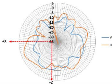
XZ-plane 6325 MHz
