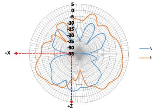
XZ-plane 6000 MHz
