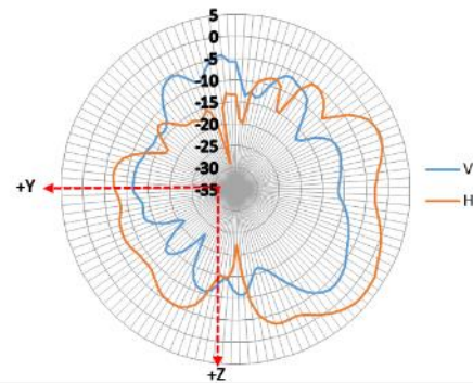
YZ-plane 5925 MHz
