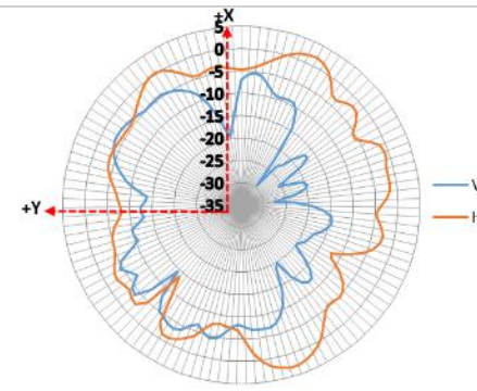
XY-plane 6925 MHz
