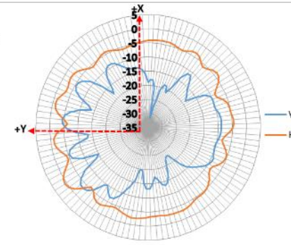
XY-plane 6225 MHz
