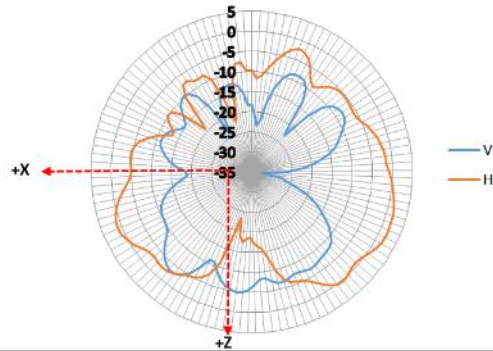
XZ-plane 5925 MHz
