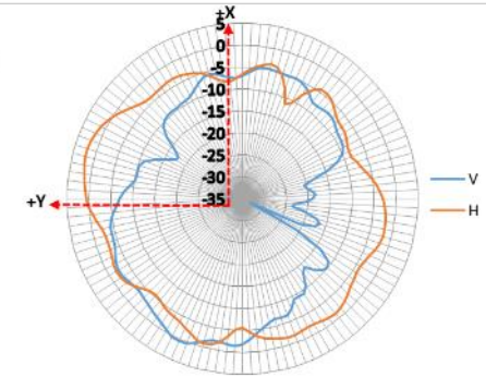
XY-plane 5150 MHz
