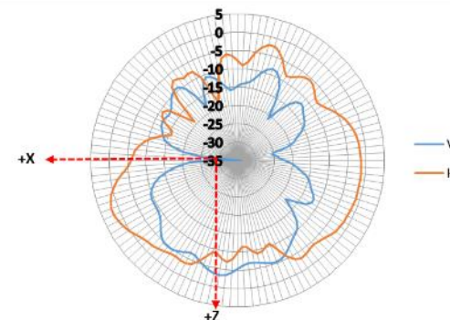
XZ-plane 6125 MHz
