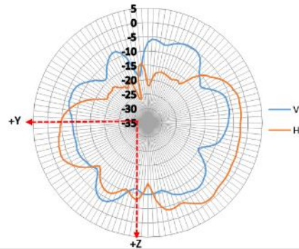
YZ-plane 6425 MHz
