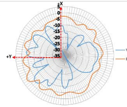
XY-plane 6325 MHz
