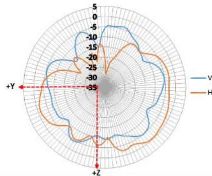
YZ-plane 6325 MHz
