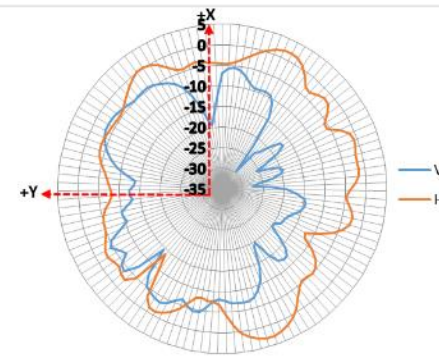
XY-plane 6875 MHz
