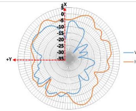
XY-plane 7000 MHz
