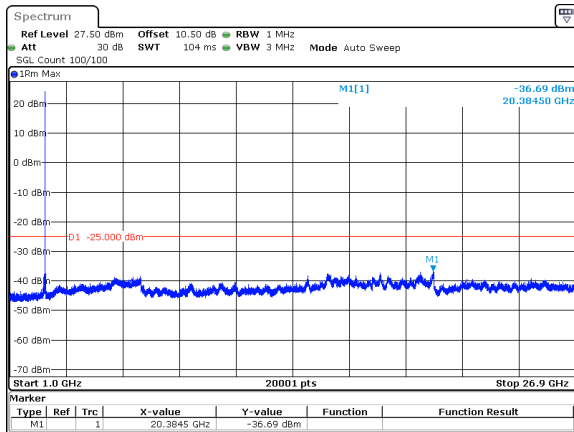
40MHz_15kHz_2593.005MHz_DFT-s-OFDM QPSK_RB1@215&amp;-36.69 dBm
