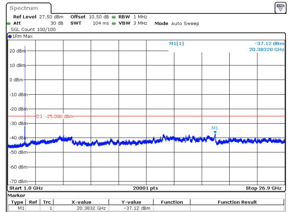
30MHz_15kHz_2593.005MHz_DFT-s-OFDM QPSK_RB1@159&amp;-37.12 dBm
