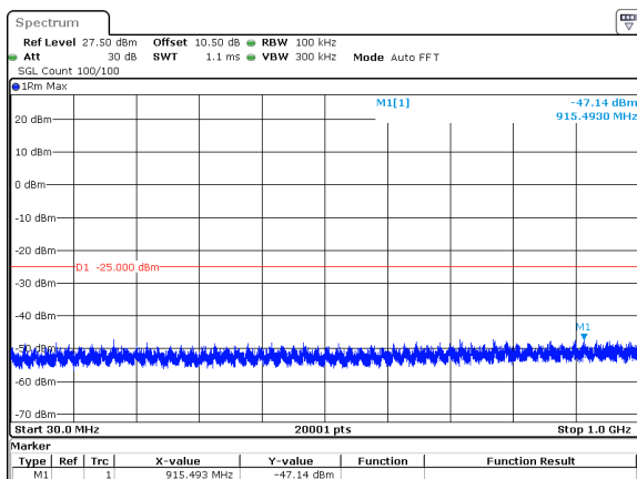
20MHz_30kHz_2679.99MHz_DFT-s-OFDM QPSK_RB50@0&amp;-47.14 dBm
