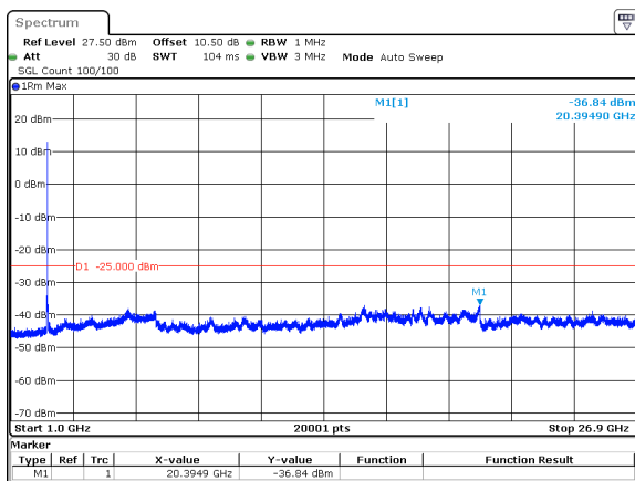
20MHz_30kHz_2506.02MHz_DFT-s-OFDM QPSK_RB50@0&amp;-36.84 dBm
