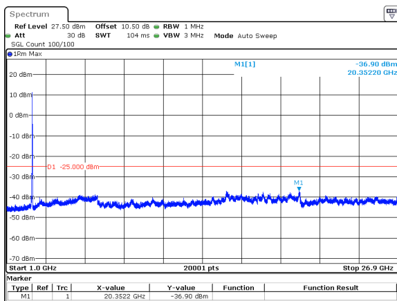
30MHz_30kHz_2674.98MHz_DFT-s-OFDM QPSK_RB75@0&amp;-36.90 dBm
