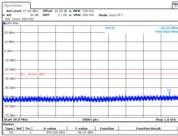
20MHz_15kHz_2593.005MHz_DFT-s-OFDM QPSK_RB1@0&amp;-46.54 dBm
