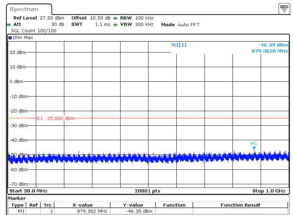
20MHz_30kHz_2592.99MHz_DFT-s-OFDM QPSK_RB1@50&amp;-46.39 dBm
