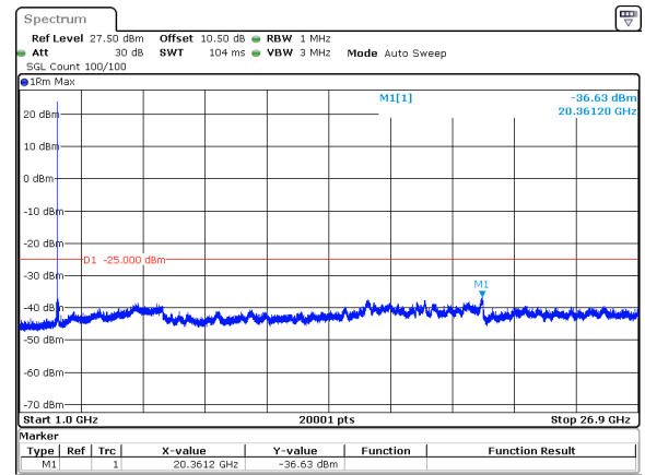
40MHz_15kHz_2593.005MHz_DFT-s-OFDM QPSK_RB1@0&amp;-36.63 dBm
