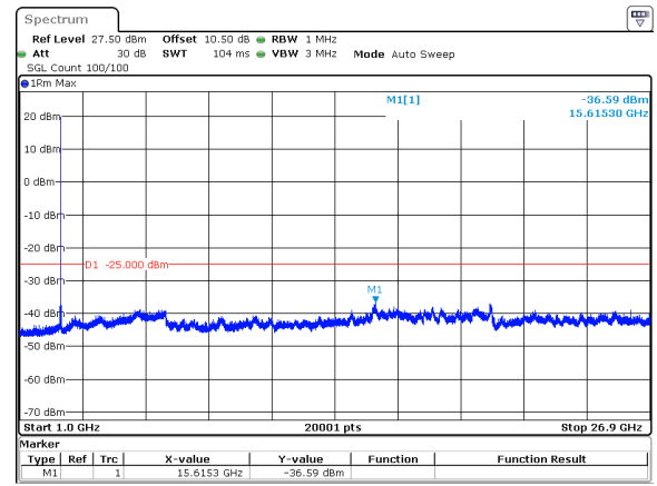
30MHz_30kHz_2674.98MHz_DFT-s-OFDM QPSK_RB1@0&amp;-36.59 dBm
