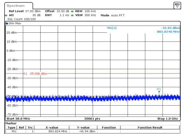
20MHz_15kHz_2593.005MHz_DFT-s-OFDM QPSK_RB100@0&amp;-45.94 dBm
