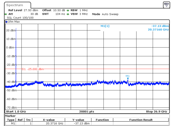
40MHz_15kHz_2670MHz_DFT-s-OFDM QPSK_RB1@215&amp;-37.13 dBm
