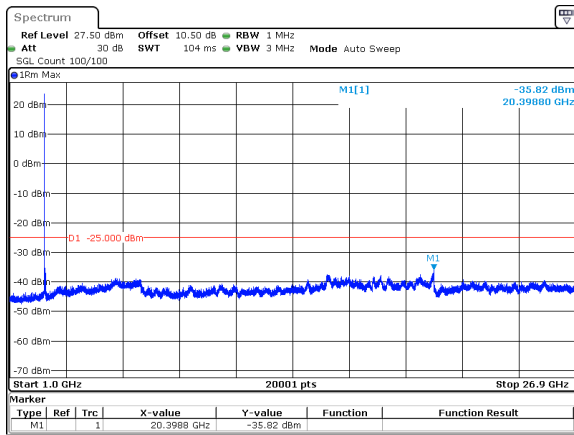
30MHz_15kHz_2593.005MHz_DFT-s-OFDM QPSK_RB1@0&amp;-35.82 dBm
