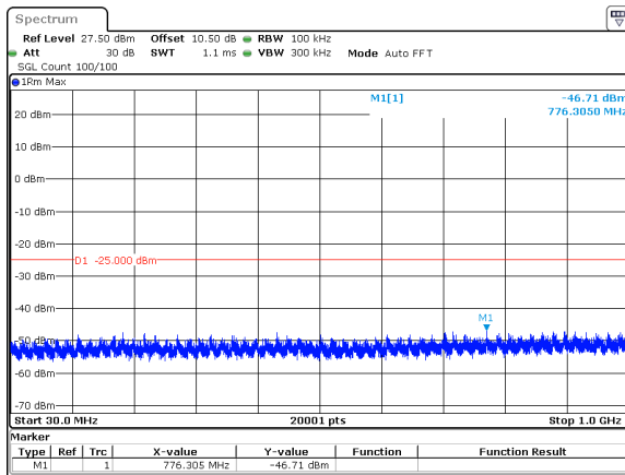
10MHz_30kHz_2685MHz_DFT-s-OFDM QPSK_RB1@23&amp;-46.71 dBm
