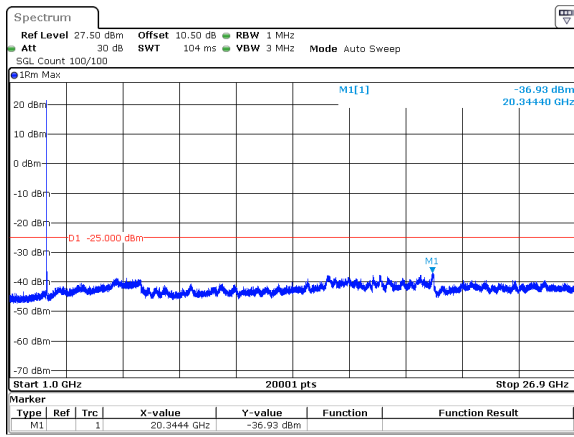
15MHz_30kHz_2682.48MHz_DFT-s-OFDM QPSK_RB1@0&amp;-36.93 dBm
