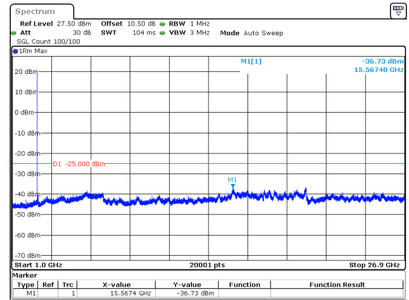
40MHz_15kHz_2670MHz_DFT-s-OFDM QPSK_RB1@0&amp;-36.73 dBm
