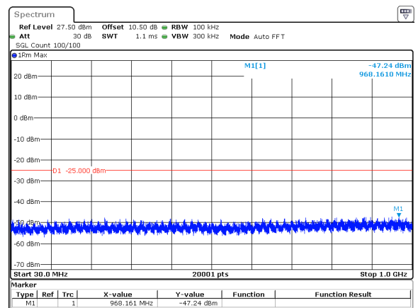
30MHz_30kHz_2592.99MHz_DFT-s-OFDM QPSK_RB75@0&amp;-47.24 dBm
