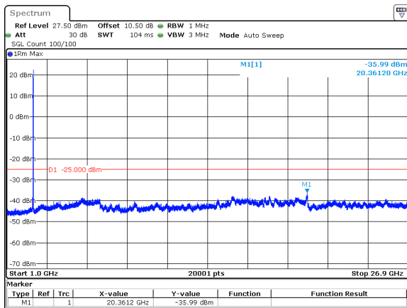
30MHz_30kHz_2674.98MHz_DFT-s-OFDM QPSK_RB1@77&amp;-35.99 dBm
