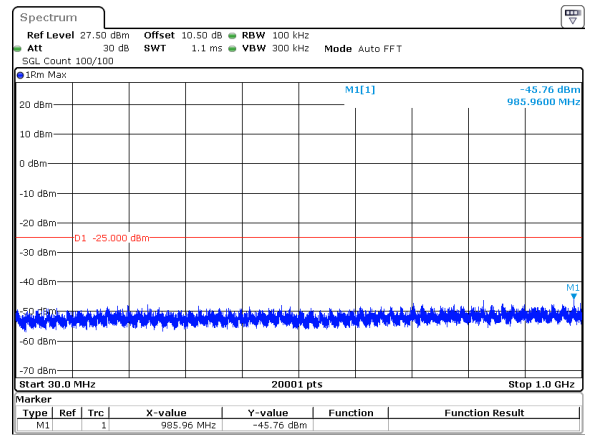
20MHz_30kHz_2679.99MHz_DFT-s-OFDM QPSK_RB1@0&amp;-45.76 dBm
