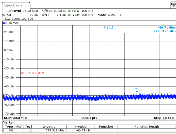
20MHz_30kHz_2592.99MHz_DFT-s-OFDM QPSK_RB1@0&amp;-46.71 dBm
