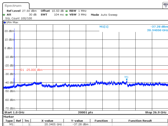
40MHz_30kHz_2670MHz_DFT-s-OFDM QPSK_RB1@105&amp;-37.28 dBm
