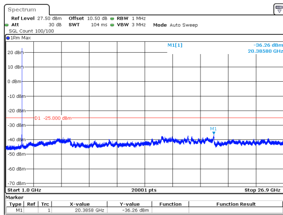
15MHz_15kHz_2503.5MHz_DFT-s-OFDM QPSK_RB1@0&amp;-36.26 dBm
