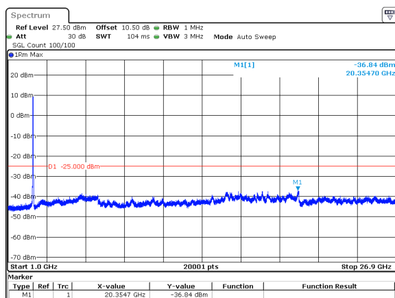
40MHz_30kHz_2670MHz_DFT-s-OFDM QPSK_RB100@0&amp;-36.84 dBm
