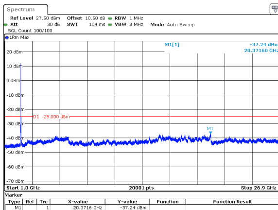
30MHz_30kHz_2511MHz_DFT-s-OFDM QPSK_RB75@0&amp;-37.24 dBm
