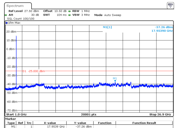
10MHz_30kHz_2685MHz_DFT-s-OFDM QPSK_RB24@0&amp;-37.26 dBm
