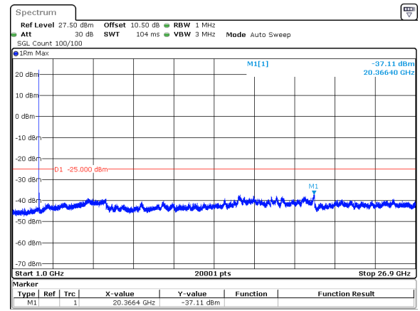
20MHz_15kHz_2679.99MHz_DFT-s-OFDM QPSK_RB1@0&amp;-37.11 dBm
