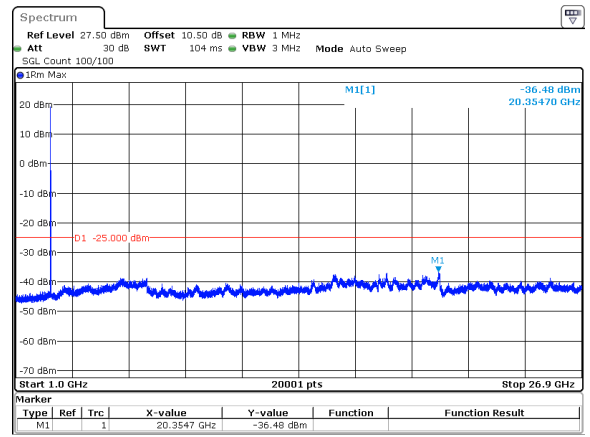
10MHz_30kHz_2592.99MHz_DFT-s-OFDM QPSK_RB1@0&amp;-36.48 dBm
