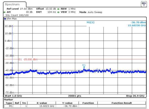
20MHz_30kHz_2506.02MHz_DFT-s-OFDM QPSK_RB1@0&amp;-36.70 dBm
