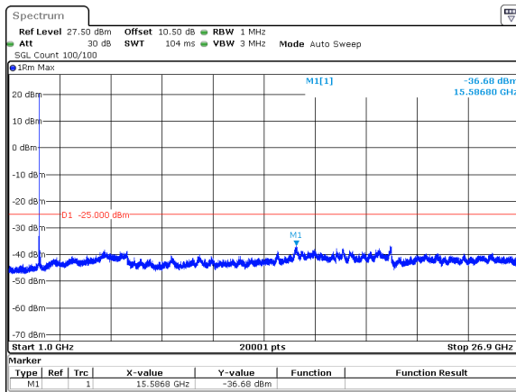
60MHz_30kHz_2526MHz_DFT-s-OFDM QPSK_RB1@161&amp;-36.68 dBm
