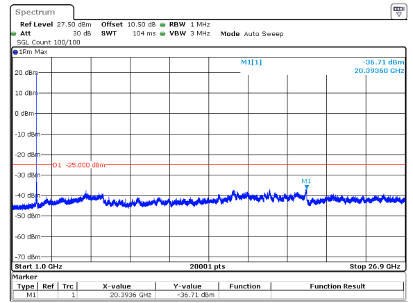
60MHz_30kHz_2592.99MHz_DFT-s-OFDM QPSK_RB1@0&amp;-36.71 dBm
