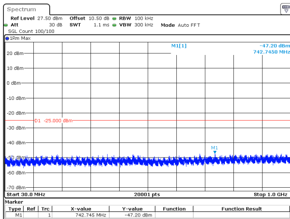
20MHz_30kHz_2506.02MHz_DFT-s-OFDM QPSK_RB1@50&amp;-47.20 dBm
