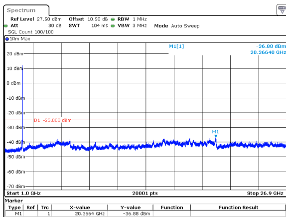
30MHz_30kHz_2592.99MHz_DFT-s-OFDM QPSK_RB75@0&amp;-36.88 dBm
