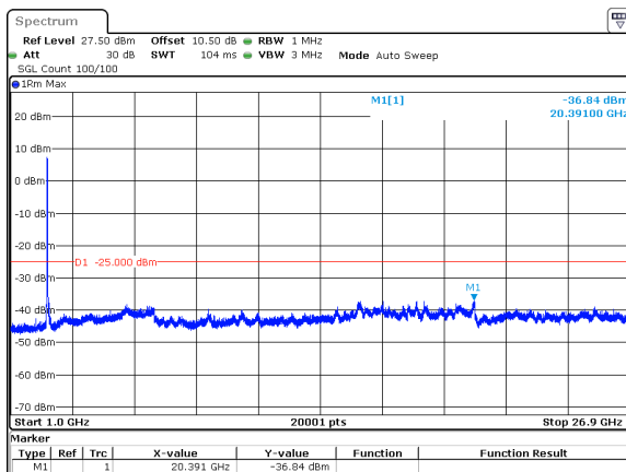
60MHz_30kHz_2526MHz_DFT-s-OFDM QPSK_RB162@0&amp;-36.84 dBm
