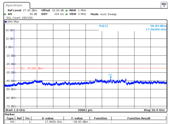
20MHz_30kHz_2506.02MHz_DFT-s-OFDM QPSK_RB1@50&amp;-36.83 dBm
