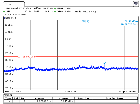
20MHz_30kHz_2592.99MHz_DFT-s-OFDM QPSK_RB1@0&amp;-36.45 dBm
