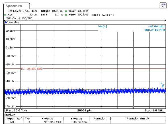
20MHz_30kHz_2592.99MHz_DFT-s-OFDM QPSK_RB50@0&amp;-46.66 dBm
