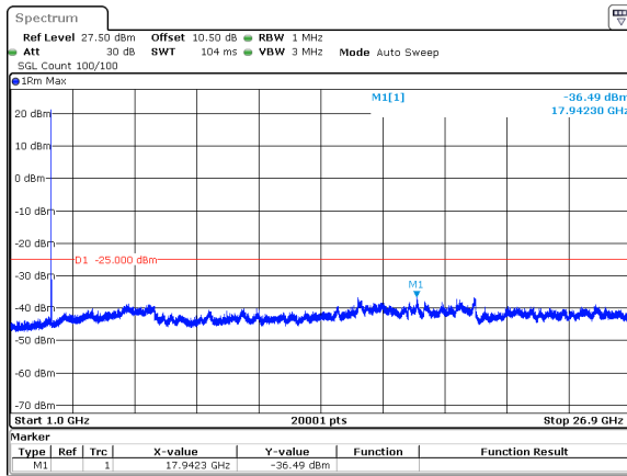
10MHz_30kHz_2685MHz_DFT-s-OFDM QPSK_RB1@0&amp;-36.49 dBm
