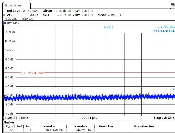
40MHz_15kHz_2670MHz_DFT-s-OFDM QPSK_RB1@215&amp;-46.70 dBm
