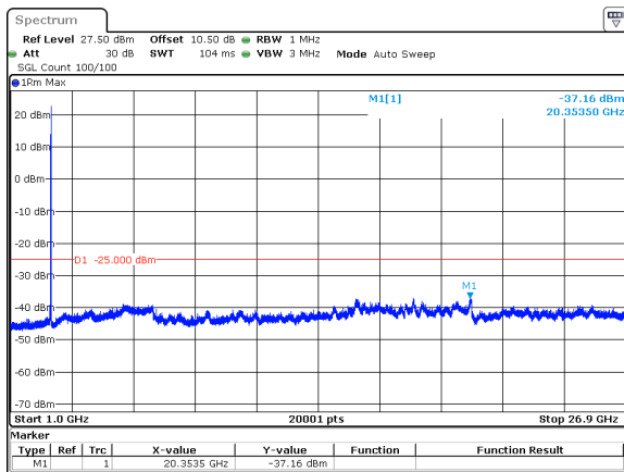
20MHz_30kHz_2679.99MHz_DFT-s-OFDM QPSK_RB1@50&amp;-37.16 dBm
