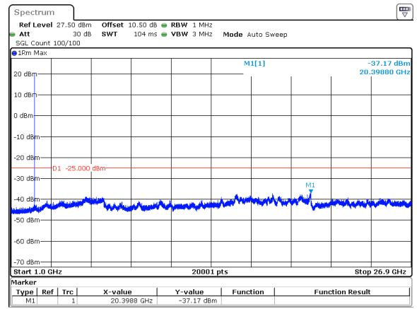
10MHz_30kHz_2501.01MHz_DFT-s-OFDM QPSK_RB1@0&amp;-37.17 dBm
