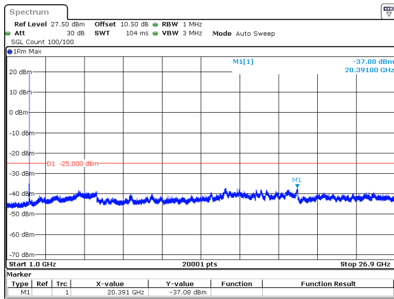
15MHz_30kHz_2503.5MHz_DFT-s-OFDM QPSK_RB1@0&amp;-37.08 dBm
