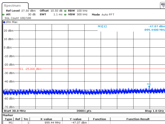
10MHz_30kHz_2685MHz_DFT-s-OFDM QPSK_RB24@0&amp;-47.07 dBm
