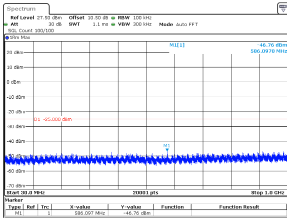
20MHz_15kHz_2506.005MHz_DFT-s-OFDM QPSK_RB1@0&amp;-46.76 dBm
