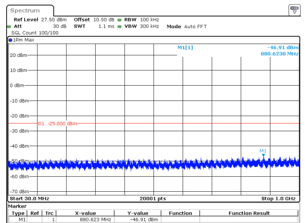
20MHz_30kHz_2506.02MHz_DFT-s-OFDM QPSK_RB50@0&amp;-46.91 dBm
