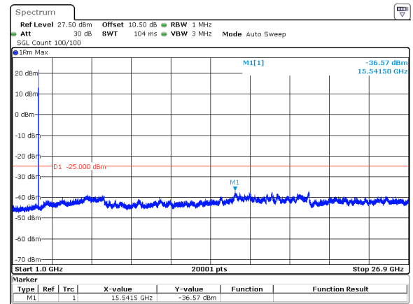
10MHz_30kHz_2685MHz_DFT-s-OFDM QPSK_RB1@23&amp;-36.57 dBm
