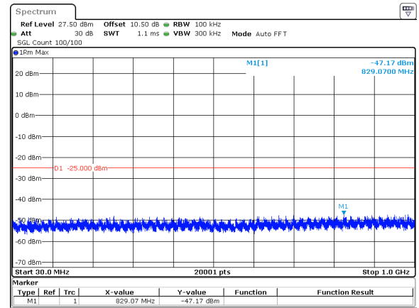
10MHz_30kHz_2685MHz_DFT-s-OFDM QPSK_RB1@0&amp;-47.17 dBm
