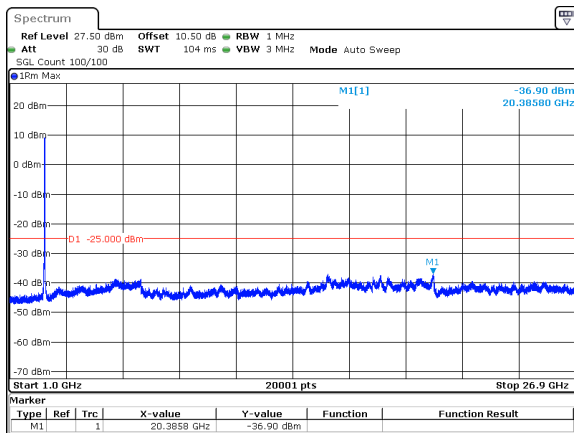
40MHz_15kHz_2593.005MHz_DFT-s-OFDM QPSK_RB216@0&amp;-36.90 dBm
