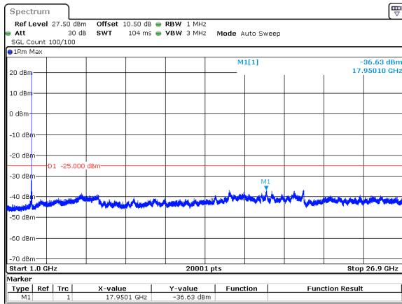
50MHz_15kHz_2593.005MHz_DFT-s-OFDM QPSK_RB1@269&amp;-36.63 dBm
