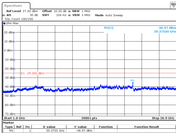
20MHz_30kHz_2592.99MHz_DFT-s-OFDM QPSK_RB1@50&amp;-36.97 dBm
