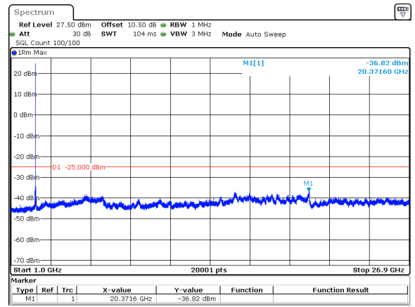
50MHz_15kHz_2593.005MHz_DFT-s-OFDM QPSK_RB1@0&amp;-36.82 dBm
