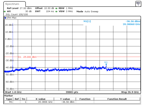
20MHz_15kHz_2593.005MHz_DFT-s-OFDM QPSK_RB1@105&amp;-36.56 dBm
