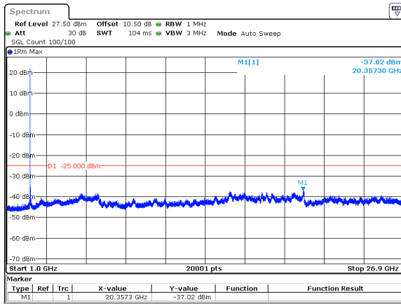
60MHz_30kHz_2526MHz_DFT-s-OFDM QPSK_RB1@0&amp;-37.02 dBm
