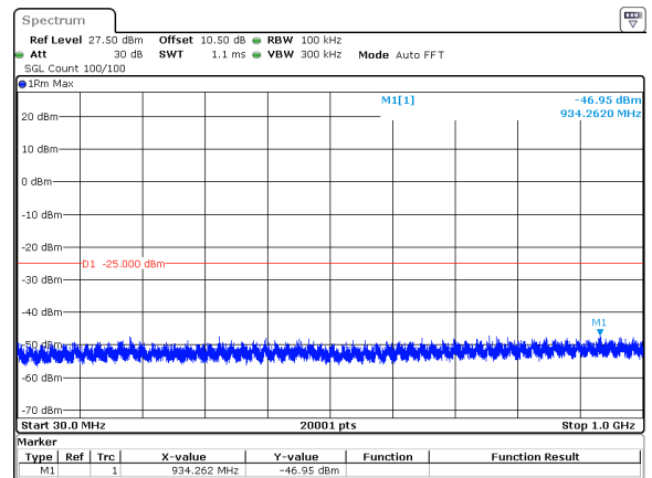
10MHz_30kHz_2501.01MHz_DFT-s-OFDM QPSK_RB24@0&amp;-46.95 dBm
