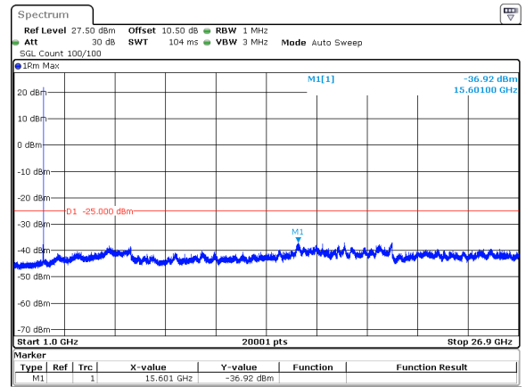
10MHz_30kHz_2501.01MHz_DFT-s-OFDM QPSK_RB1@23&amp;-36.92 dBm
