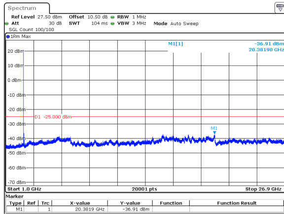
40MHz_30kHz_2670MHz_DFT-s-OFDM QPSK_RB1@0&amp;-36.91 dBm
