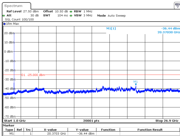
10MHz_30kHz_2592.99MHz_DFT-s-OFDM QPSK_RB1@23&amp;-36.44 dBm
