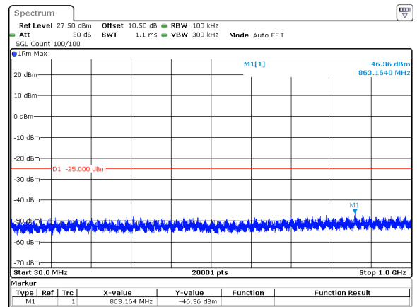
20MHz_30kHz_2679.99MHz_DFT-s-OFDM QPSK_RB1@50&amp;-46.36 dBm
