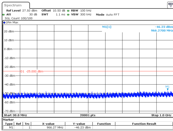
30MHz_30kHz_2674.98MHz_DFT-s-OFDM QPSK_RB1@0&amp;-46.23 dBm
