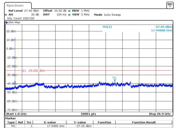
20MHz_15kHz_2506.005MHz_DFT-s-OFDM QPSK_RB100@0&amp;-37.05 dBm
