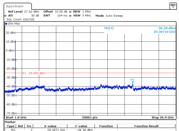
30MHz_15kHz_2593.005MHz_DFT-s-OFDM QPSK_RB160@0&amp;-36.38 dBm
