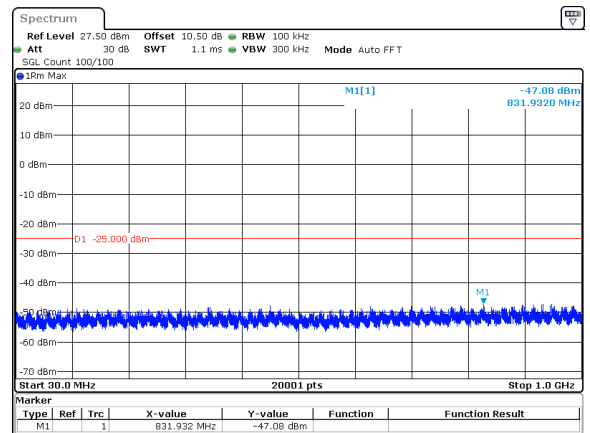
50MHz_15kHz_2593.005MHz_DFT-s-OFDM QPSK_RB270@0&amp;-47.08 dBm
