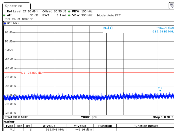
40MHz_15kHz_2670MHz_DFT-s-OFDM QPSK_RB216@0&amp;-46.14 dBm
