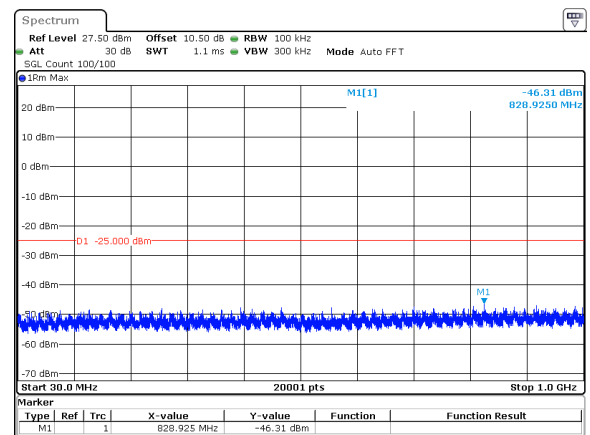
30MHz_30kHz_2674.98MHz_DFT-s-OFDM QPSK_RB75@0&amp;-46.31 dBm
