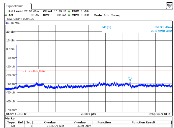
20MHz_15kHz_2679.99MHz_DFT-s-OFDM QPSK_RB100@0&amp;-36.91 dBm
