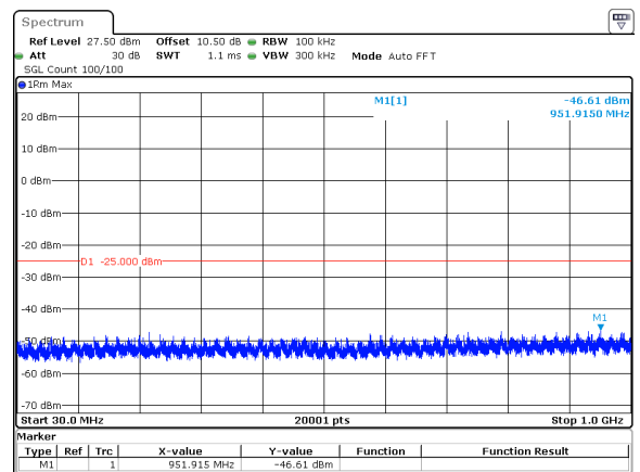
10MHz_30kHz_2592.99MHz_DFT-s-OFDM QPSK_RB24@0&amp;-46.61 dBm
