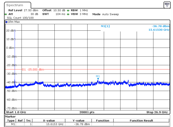
20MHz_15kHz_2506.005MHz_DFT-s-OFDM QPSK_RB1@0&amp;-36.78 dBm
