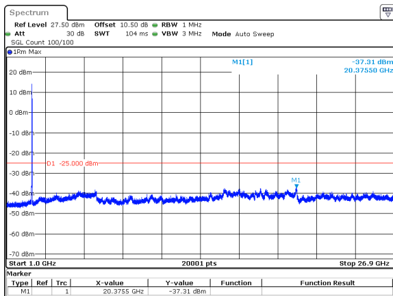
15MHz_30kHz_2682.48MHz_DFT-s-OFDM QPSK_RB36@0&amp;-37.31 dBm
