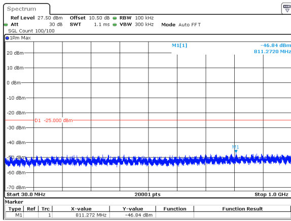
20MHz_30kHz_2506.02MHz_DFT-s-OFDM QPSK_RB1@0&amp;-46.84 dBm
