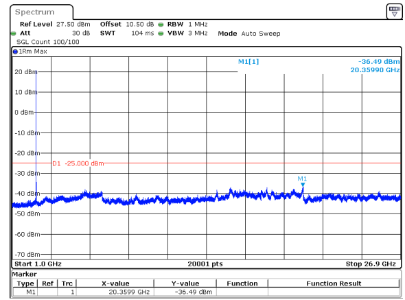
20MHz_15kHz_2593.005MHz_DFT-s-OFDM QPSK_RB1@0&amp;-36.49 dBm
