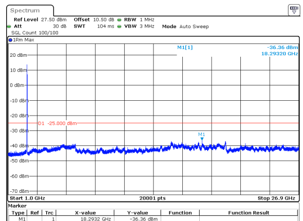
20MHz_30kHz_2679.99MHz_DFT-s-OFDM QPSK_RB50@0&amp;-36.36 dBm
