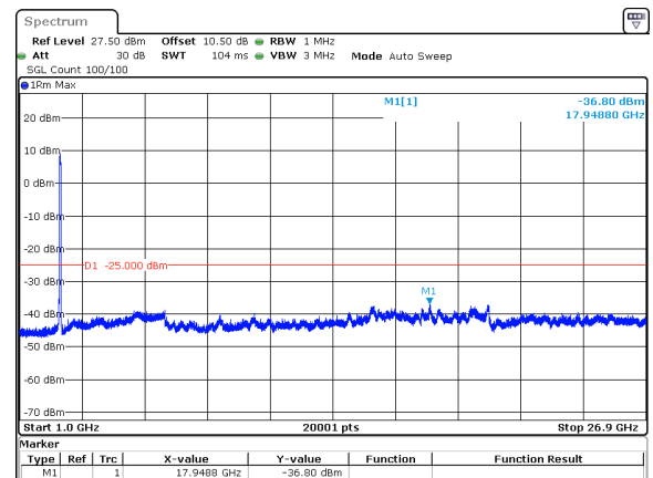
40MHz_15kHz_2670MHz_DFT-s-OFDM QPSK_RB216@0&amp;-36.80 dBm
