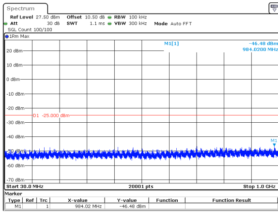
20MHz_15kHz_2679.99MHz_DFT-s-OFDM QPSK_RB1@0&amp;-46.48 dBm
