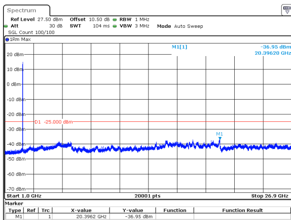
10MHz_30kHz_2592.99MHz_DFT-s-OFDM QPSK_RB24@0&amp;-36.95 dBm
