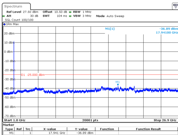
20MHz_30kHz_2592.99MHz_DFT-s-OFDM QPSK_RB50@0&amp;-36.89 dBm
