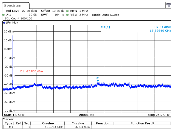
10MHz_30kHz_2501.01MHz_DFT-s-OFDM QPSK_RB24@0&amp;-37.04 dBm
