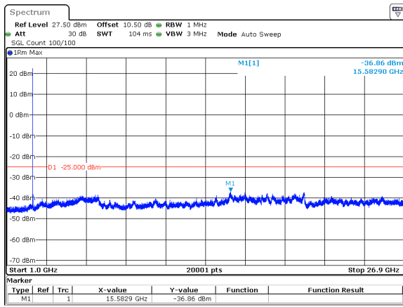
20MHz_30kHz_2679.99MHz_DFT-s-OFDM QPSK_RB1@0&amp;-36.86 dBm
