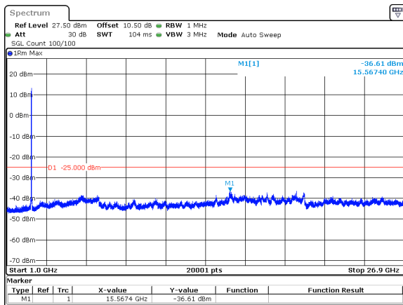
20MHz_15kHz_2593.005MHz_DFT-s-OFDM QPSK_RB100@0&amp;-36.61 dBm
