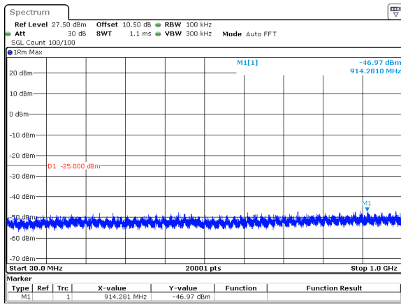
10MHz_30kHz_2501.01MHz_DFT-s-OFDM QPSK_RB1@0&amp;-46.97 dBm
