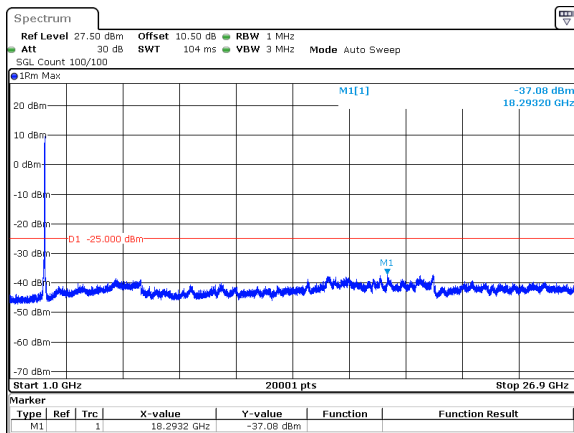
50MHz_15kHz_2593.005MHz_DFT-s-OFDM QPSK_RB270@0&amp;-37.08 dBm
