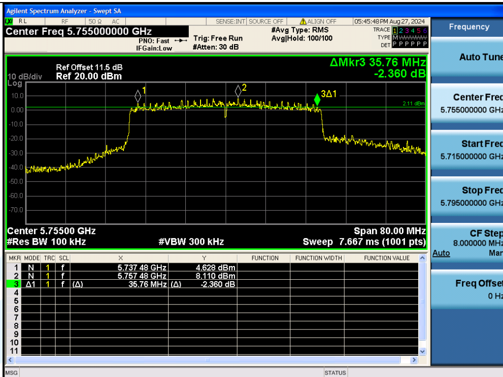
11AX40MIMO-Ant3-5755-PASS
