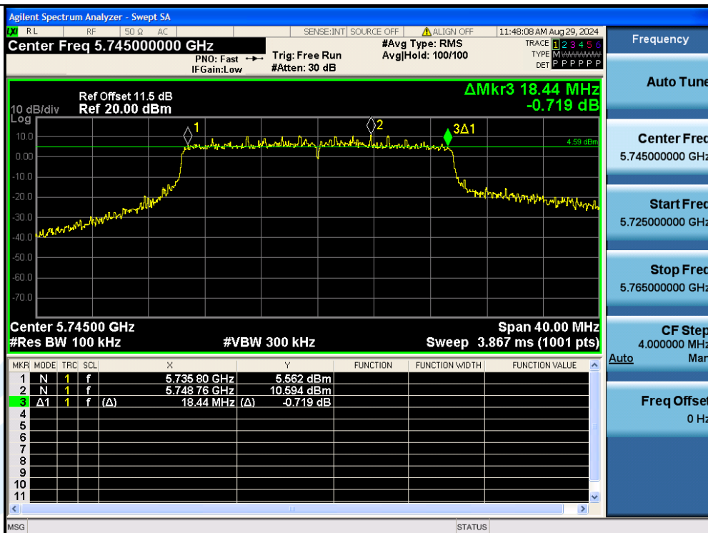
11AX20MIMO-Ant3-5745-PASS
