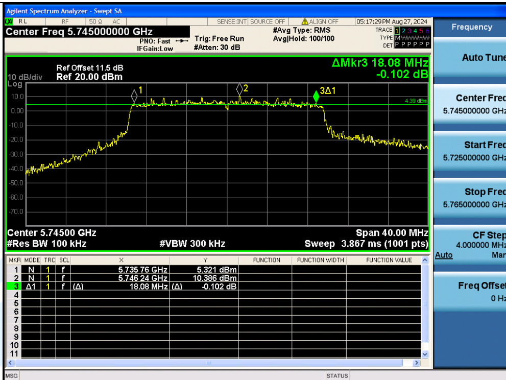
11AX20MIMO-Ant3-5745-PASS
