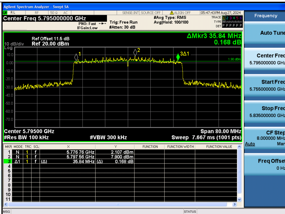
11AX40MIMO-Ant3-5795-PASS
