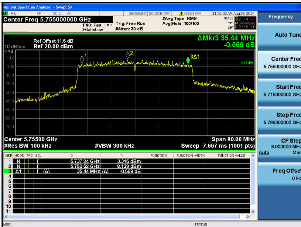
11AX40MIMO-Ant3-5755-PASS
