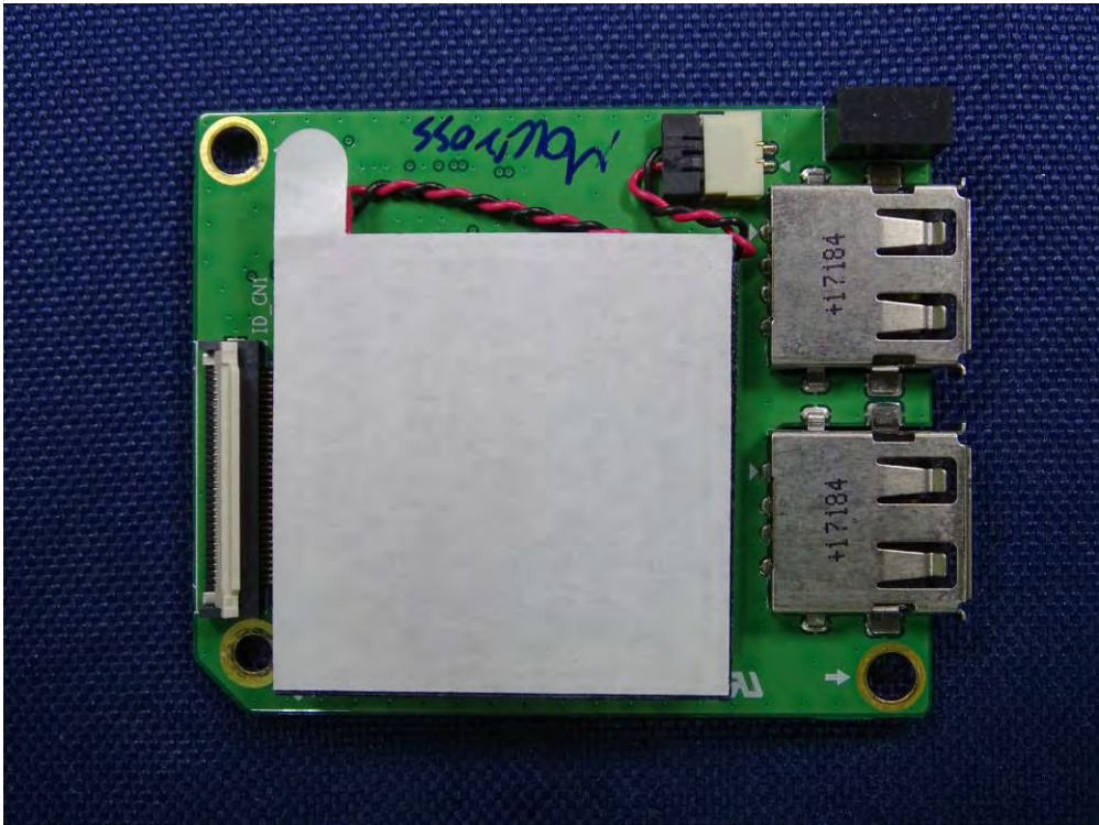
(17) EUT Photo - NFC
