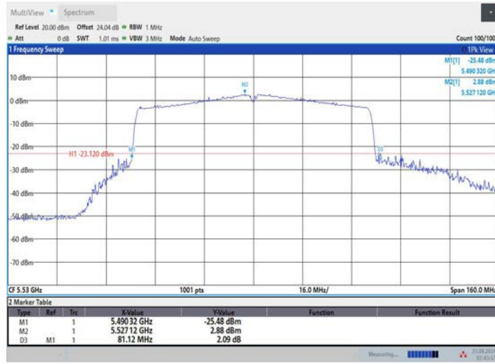
11AC80MIMO_Ant2_5530
