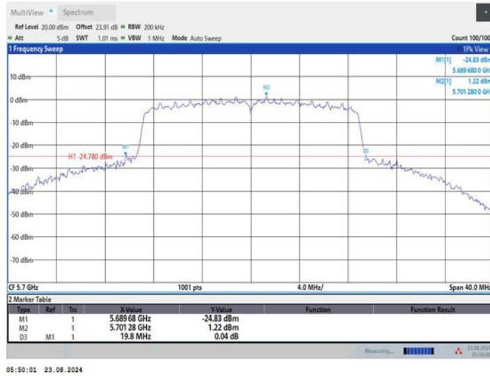
11AC20MIMO_Ant3_5700
