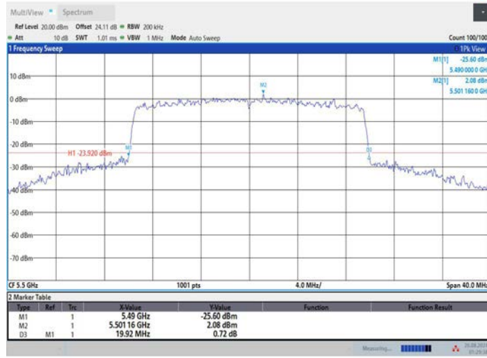
11AX20MIMO_Ant3_5500
