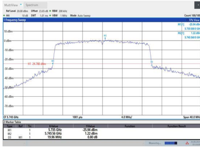
11AX20MIMO_Ant2_5745
