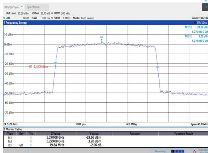
11AX20MIMO_Ant2_5280
