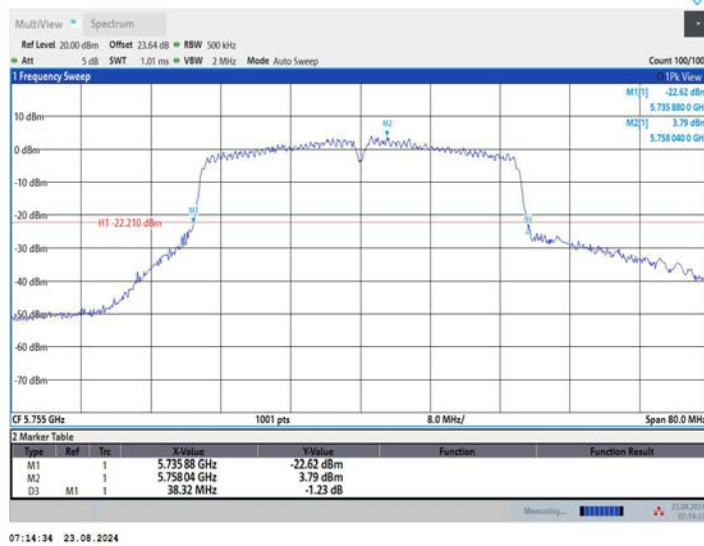
11AC40MIMO_Ant3_5755
