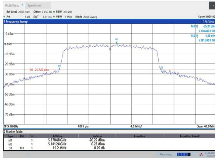
11AC20MIMO_Ant3_5180
