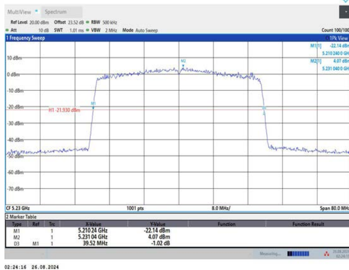
11AX40MIMO_Ant3_5230
