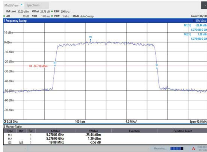
11AX20MIMO_Ant3_5280
