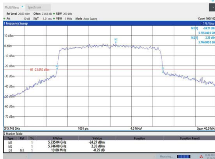
11AX20MIMO_Ant3_5745
