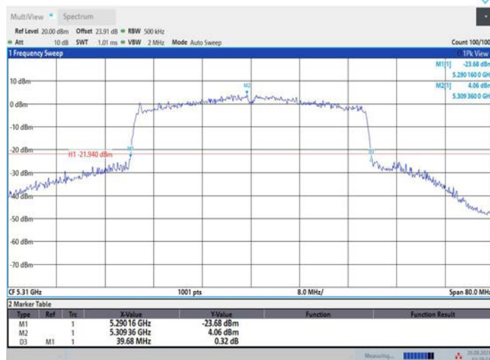
11AX40MIMO_Ant3_5310
