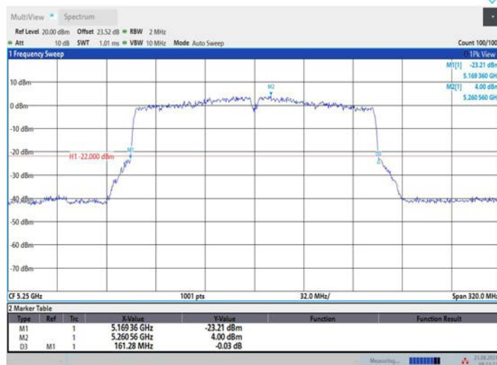
11AC160MIMO_Ant2_5250
