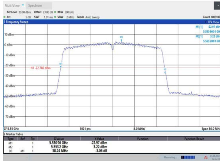
11N40MIMO_Ant3_5550
