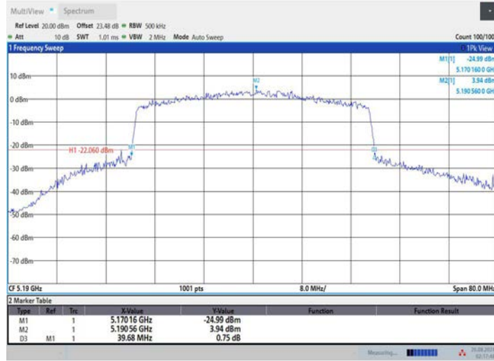
11AX40MIMO_Ant3_5190
