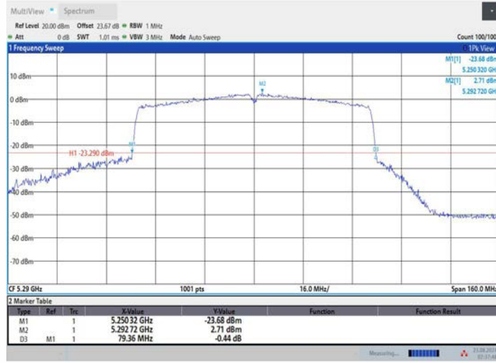
11AC80MIMO_Ant3_5290
