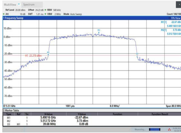
11AX40MIMO_Ant3_5510
