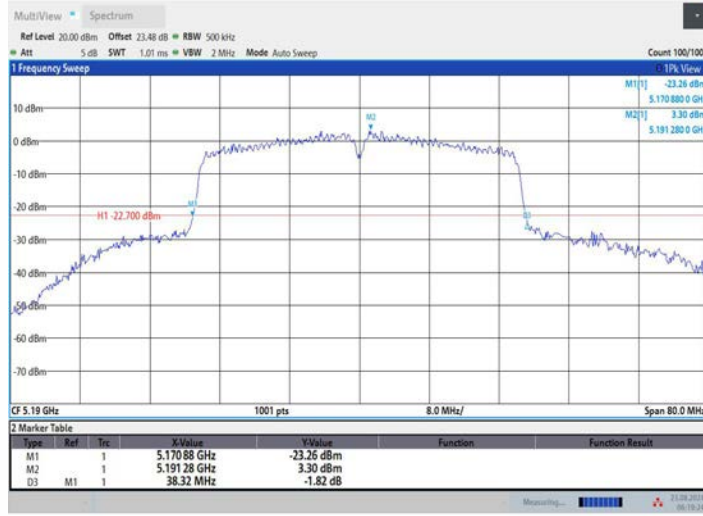
11AC40MIMO_Ant3_5190
