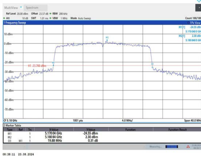
11AX20MIMO_Ant2_5180
