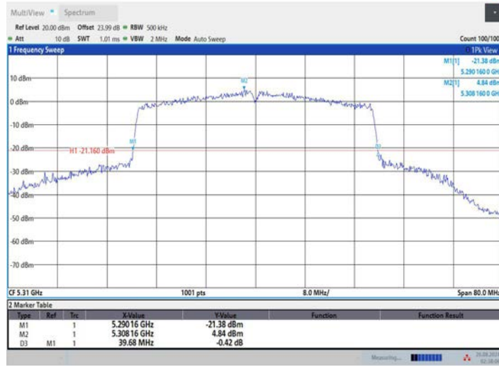
11AX40MIMO_Ant2_5310
