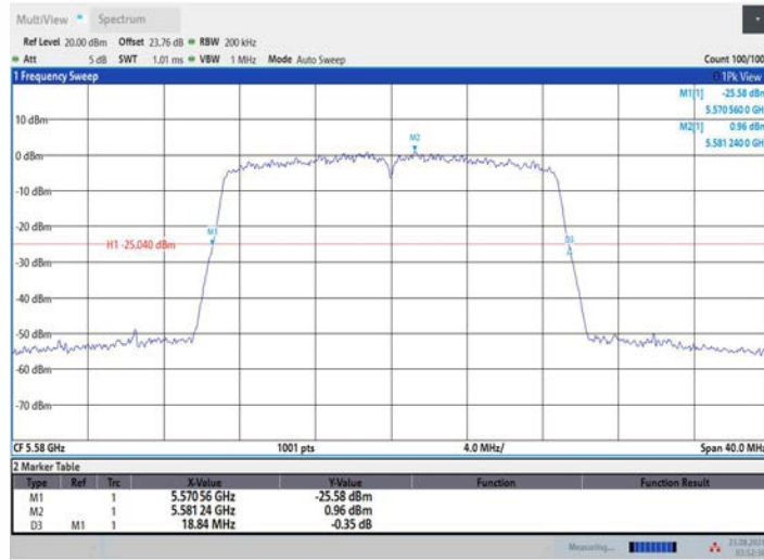
11AC20MIMO_Ant2_5580
