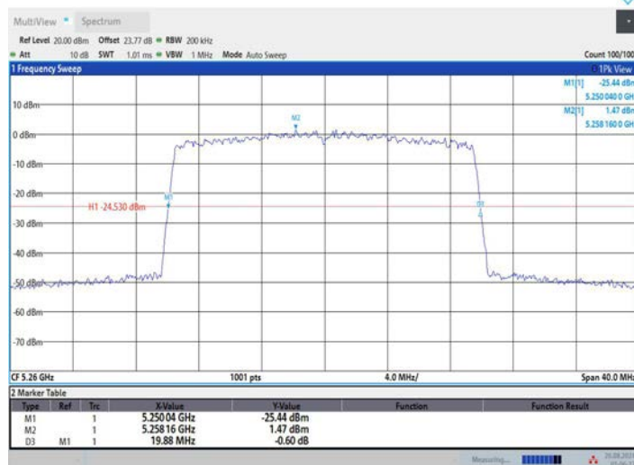
11AX20MIMO_Ant3_5260
