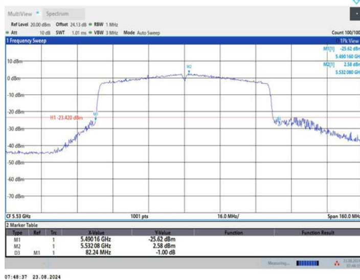
11AC80MIMO_Ant3_5530
