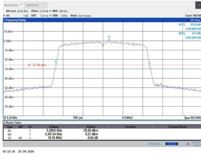
11AC20MIMO_Ant3_5240
