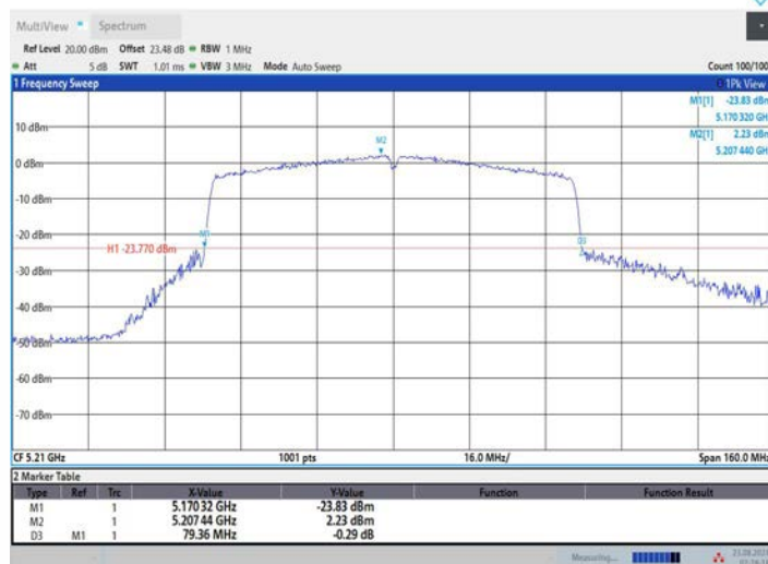
11AC80MIMO_Ant3_5210
