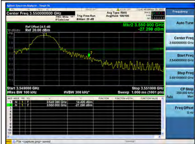
Band42 / 10MHz / High CH / QPSK / 1 RB
