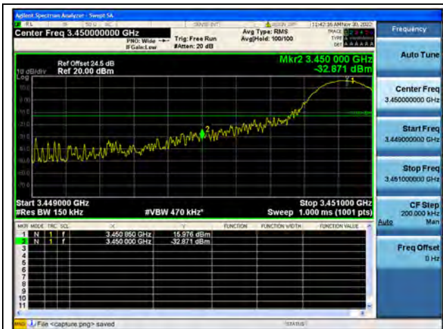
Band42 / 15MHz / Low CH / QPSK / 1 RB
