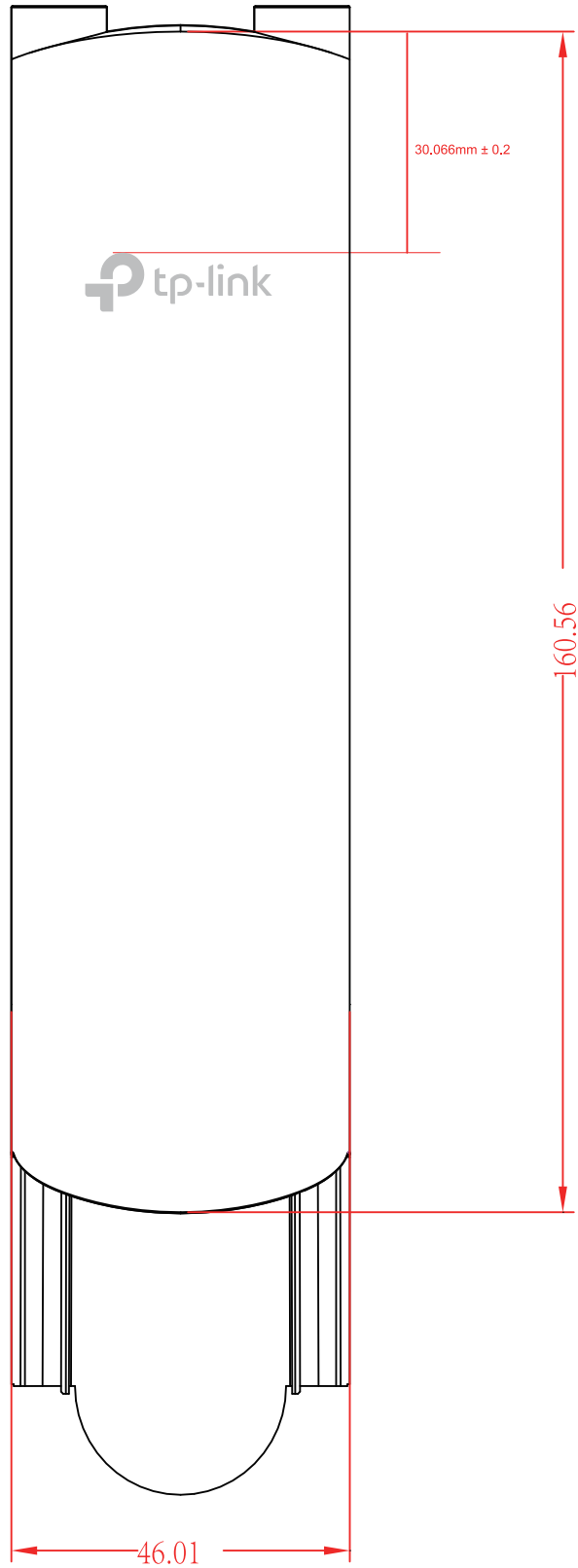
尺寸图
