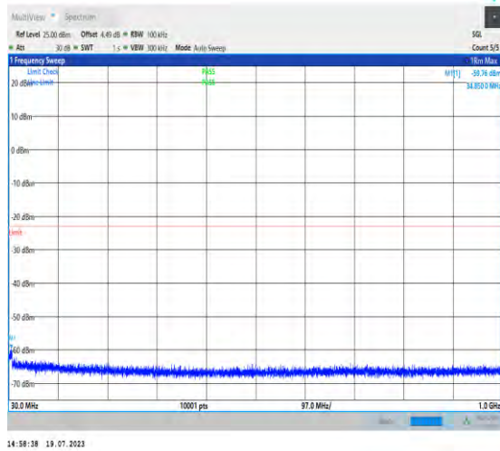
1-N66-PC3-15-40-M-1-DFT-PI2BPSK-Inner_1RB_L eft-1@1-30-1000-Ant3-34.85--59.76--23-PASS
