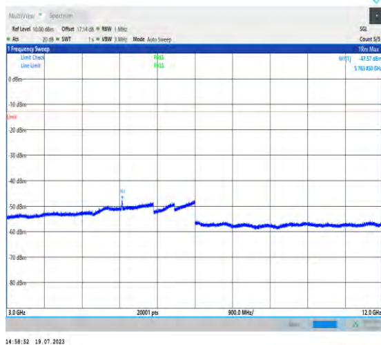
1-N66-PC3-15-40-M-1-DFT-PI2BPSK-Inner_1RB_L eft-1@1-3000-12000-Ant3-5763.45--47.57--13-PAS S
