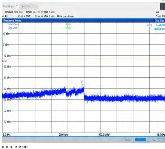
1-N66-PC3-15-40-M-1-DFT-PI2BPSK-Inner_1RB_L eft-1@1-3000-12000-Ant3-7393.80--37.52--13-PAS
