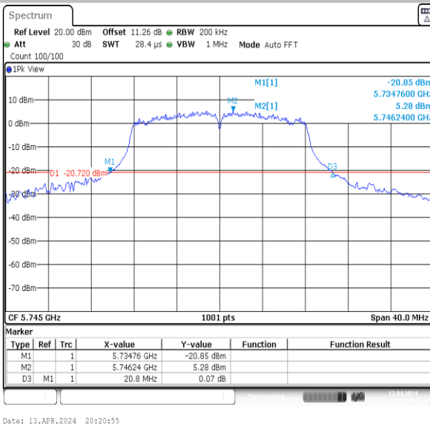
11A-Ant1-5745
