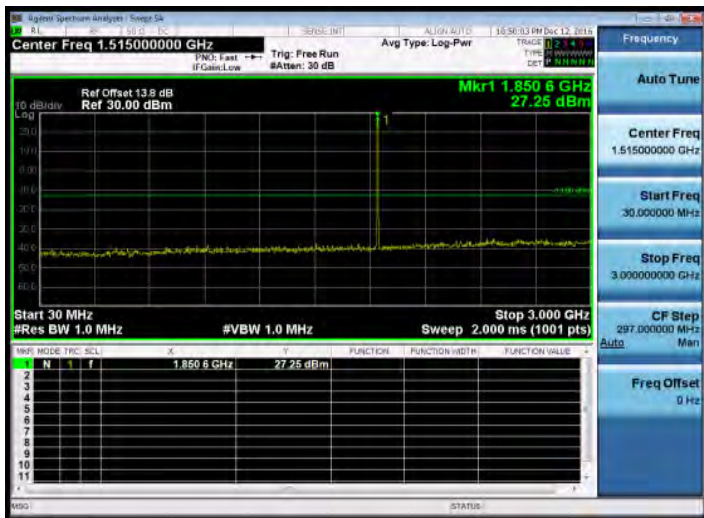
30MHz~3GHz_Band2_3MHz_QPSK_1_0_LowCH18615-1851.5
