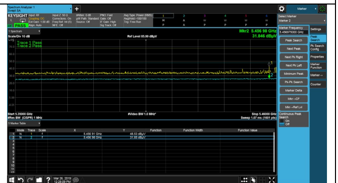
802.11n-HT20 5500M
