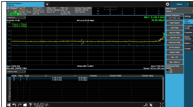
802.11a 5180M
