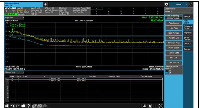
802.11a 5320M
