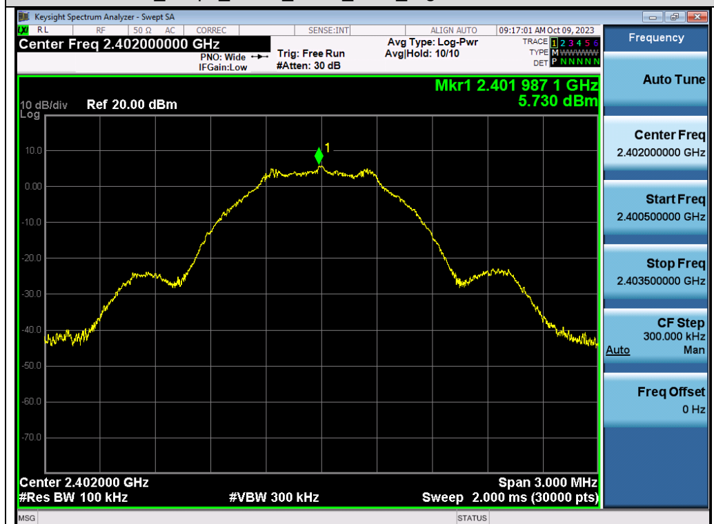
Test_Graph_GFSK_ANT2_2402_Reference Level
