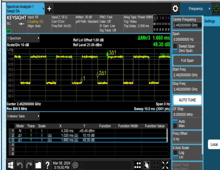
NTNV-11AX20MIMO-Ant1-2462
