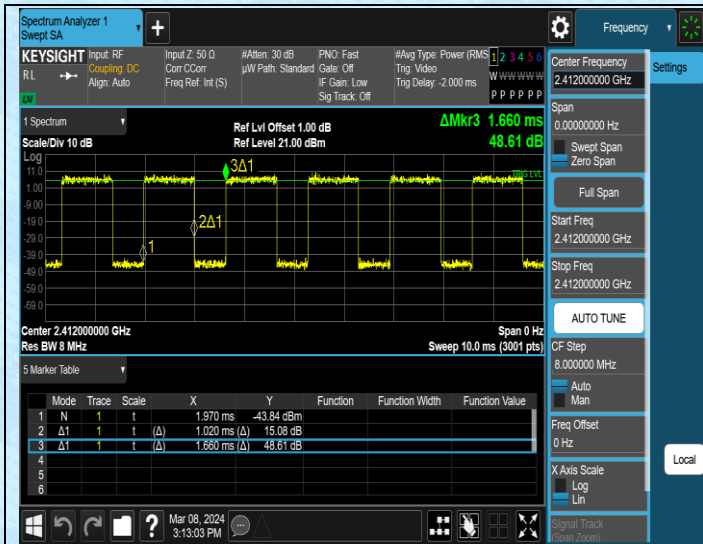
NTNV-11AX20MIMO-Ant1-2412
