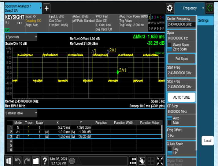
NTNV-11AX20MIMO-Ant2-2437
