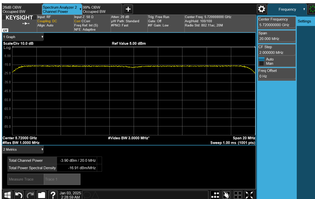
Wave-MLO5_UNII-2C_HE20_5720_CH1
