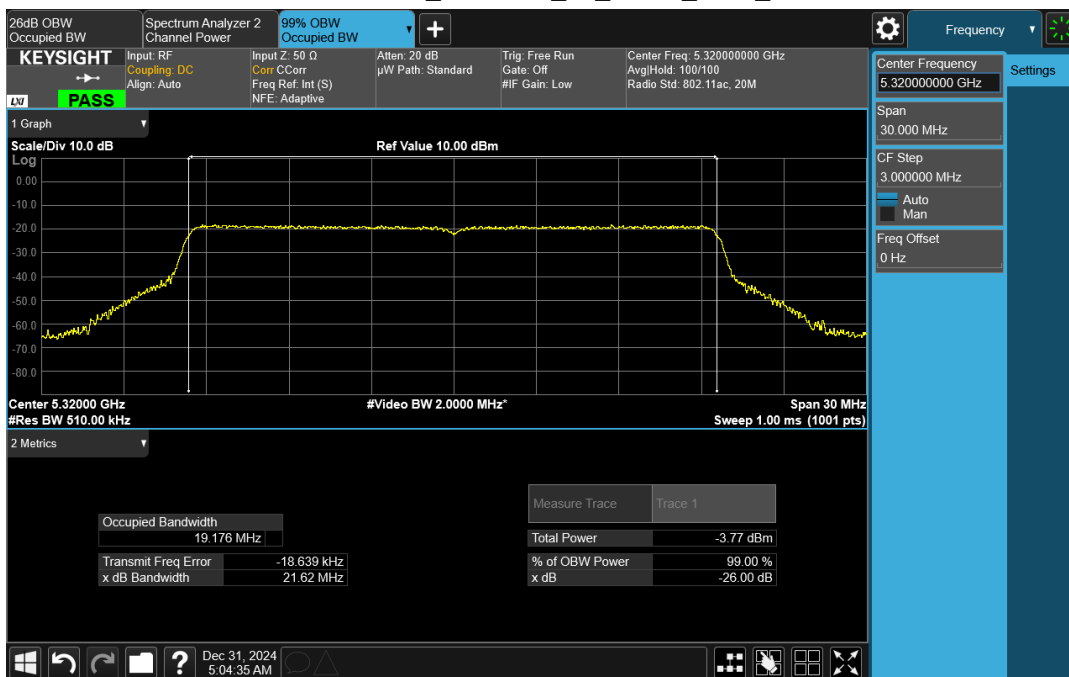
Wave-MLO5_UNII-2A_99_HE20_5320_CH0
