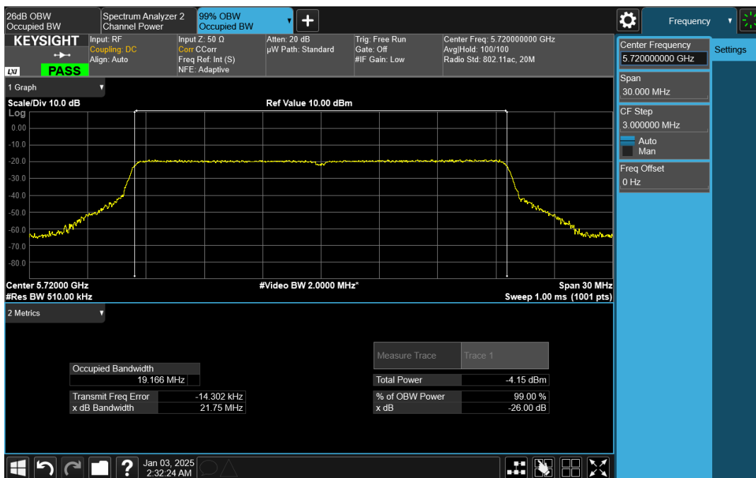
Wave-MLO5_UNII-2C_99_HE20_5720_CH0
