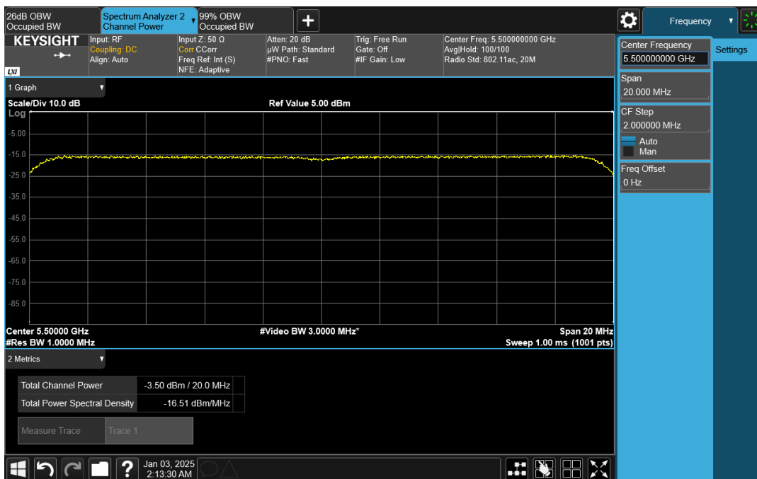
Wave-MLO5_UNII-2C_HE20_5500_CH0
