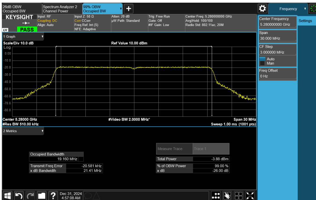
Wave-MLO5_UNII-2A_99_HE20_5280_CH0
