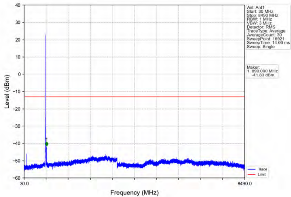
Band26b_10MHz_QPSK_HCH_844MHz_RB_1_49_NTNV
