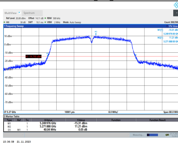
11AC40MIMO_Ant2_5270
