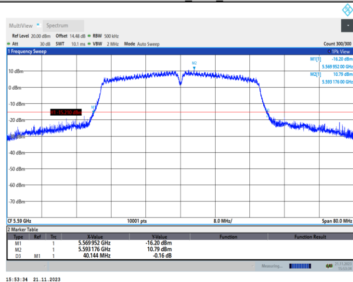
11AC40MIMO_Ant2_5590
