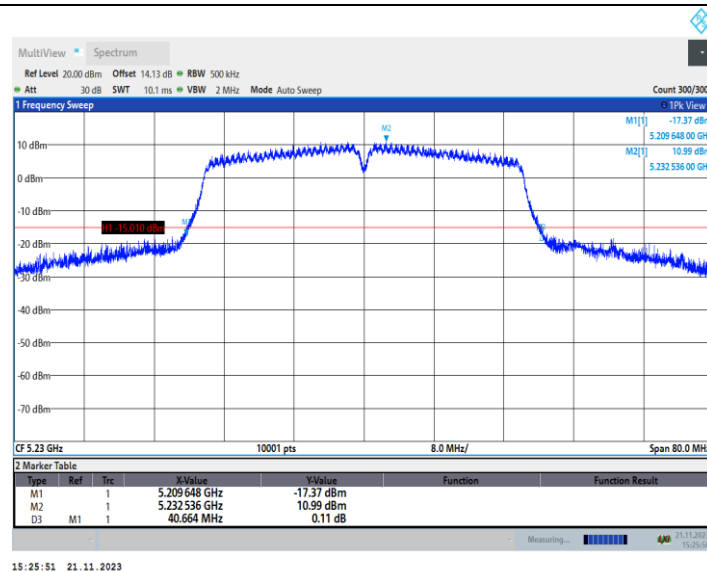
11AC40MIMO_Ant2_5230
