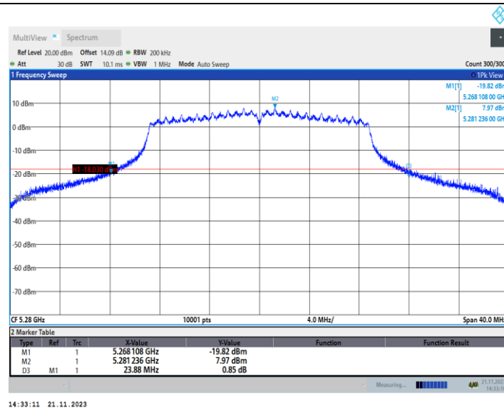
11AC20MIMO_Ant2_5280
