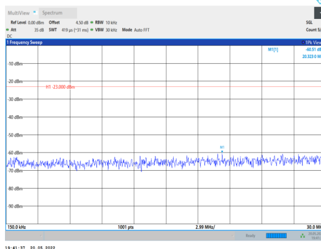
Band26-10MHz-QPSK-26740-1RB#0-Range2:0.15~30MHz
