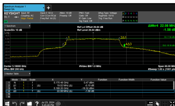
Figure 329 - 802.11ax HE20 SU Maximum 99% OBW
