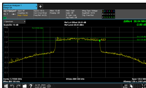
Figure 317 - 802.11ax HE40 SU Maximum 6 dB EBW
