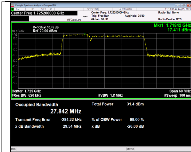
66-66-10MHz-20MHz-QPSK-QPSK-132027-132171-50RB #0-100RB#0-PASS
