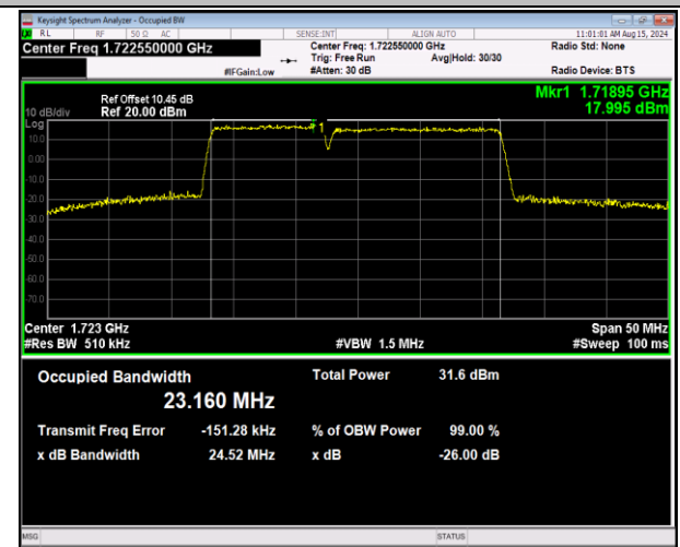
66-66-10MHz-15MHz-QPSK-QPSK-132025-132145-50RB #0-75RB#0-PASS
