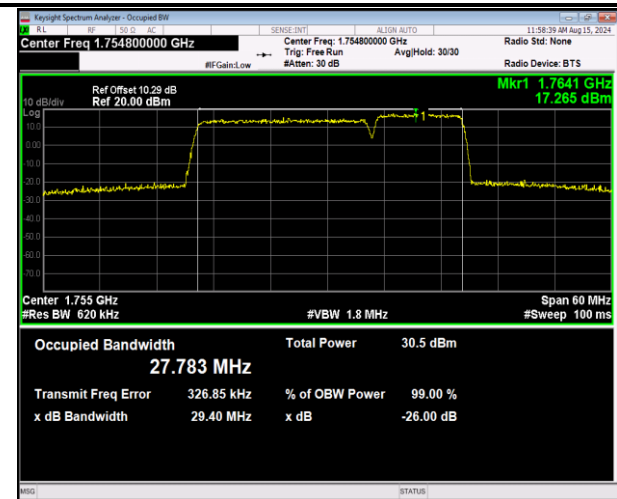
66-66-20MHz-10MHz-16QAM-16QAM-132373-132517-10 ORB#0-50RB#0-PASS
