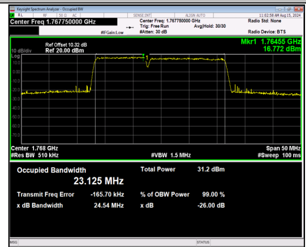
66-66-10MHz-15MHz-QPSK-QPSK-132477-132597-50RB #0-75RB#0-PASS
