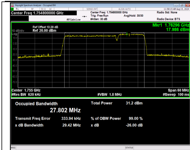
66-66-20MHz-10MHz-QPSK-QPSK-132373-132517-100R B#0-50RB#0-PASS
