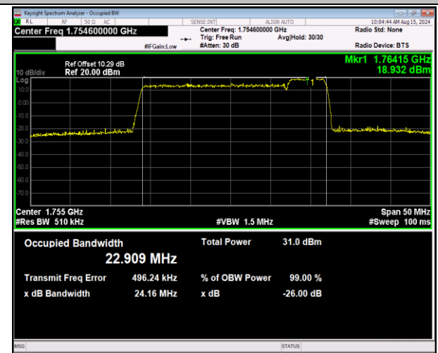
66-66-20MHz-5MHz-QPSK-QPSK-132397-132514-100RB #0-25RB#0-PASS
