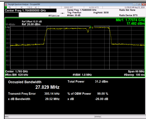
66-66-20MHz-10MHz-QPSK-QPSK-132473-132617-100R B#0-50RB#0-PASS
