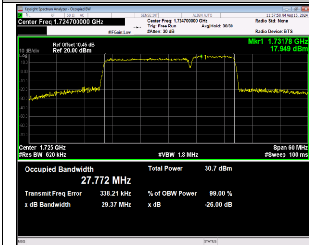
66-66-20MHz-10MHz-16QAM-16QAM-132072-132216-10ORB #0-50RB#0-PASS
