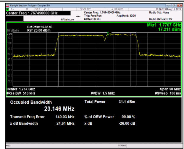
66-66-15MHz-10MHz-QPSK-QPSK-132499-132619-75RB #0-50RB#0-PASS
