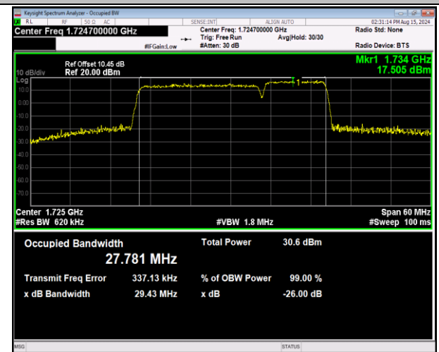
66-66-20MHz-10MHz-64QAM-64QAM-132072-132216-10ORB #0-50RB#0-PASS
