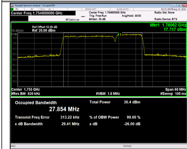
66-66-20MHz-10MHz-64QAM-64QAM-132373-132517-10 ORB#0-50RB#0-PASS
