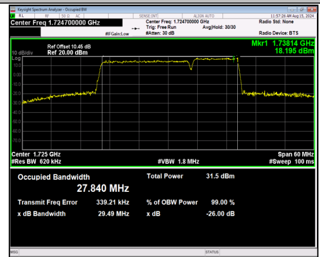
66-66-20MHz-10MHz-QPSK-QPSK-132072-132216-100RB #0-50RB#0-PASS
