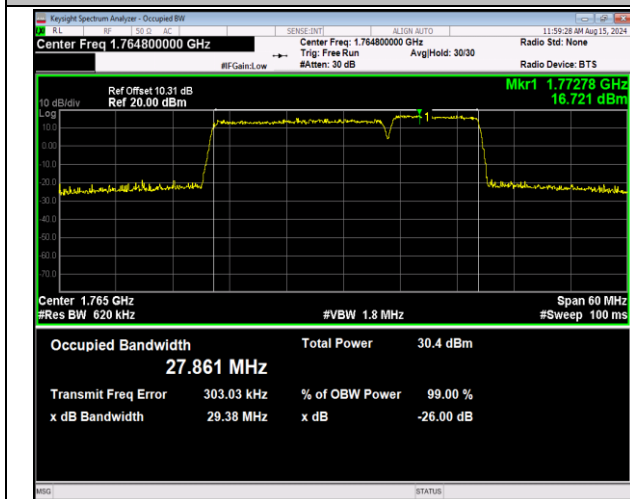
66-66-20MHz-10MHz-16QAM-16QAM-132473-132617-10 ORB#0-50RB#0-PASS
