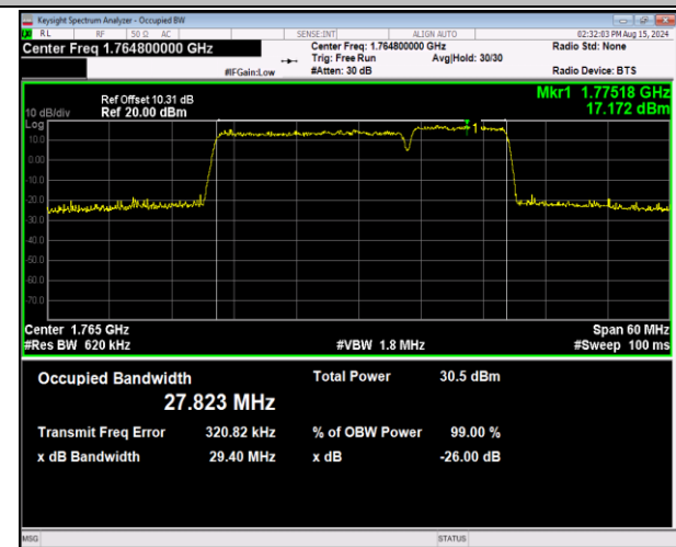
66-66-20MHz-10MHz-64QAM-64QAM-132473-132617-10 ORB#0-50RB#0-PASS
