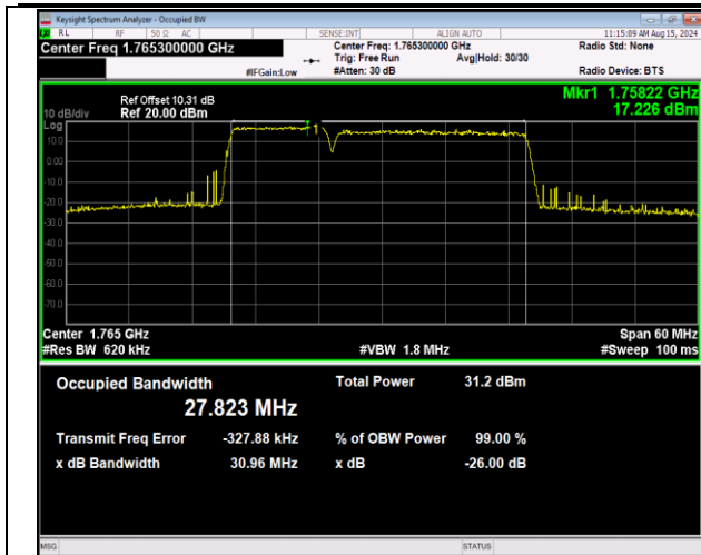
66-66-10MHz-20MHz-QPSK-QPSK-132428-132572-50RB #0-100RB#0-PASS
