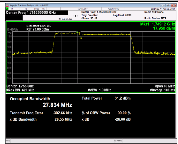
66-66-10MHz-20MHz-QPSK-QPSK-132328-132472-50RB #0-100RB#0-PASS
