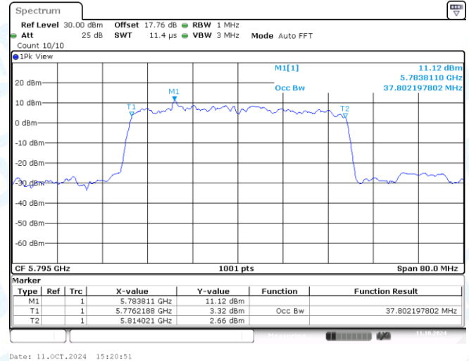
11AX40MIMO-Ant2-5795
