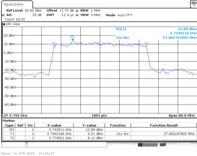
11AX40MIMO-Ant1-5755
