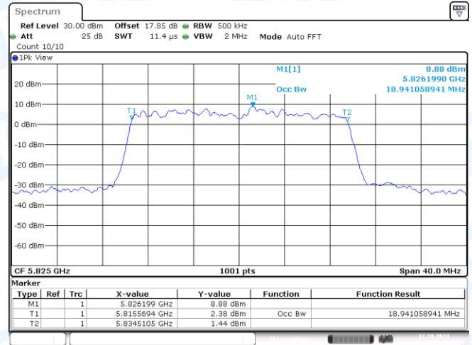
11AX20MIMO-Ant2-5825
