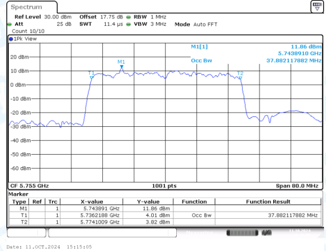
11AX40MIMO-Ant2-5755
