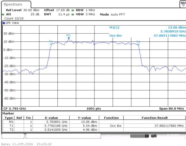
11AX40MIMO-Ant1-5795
