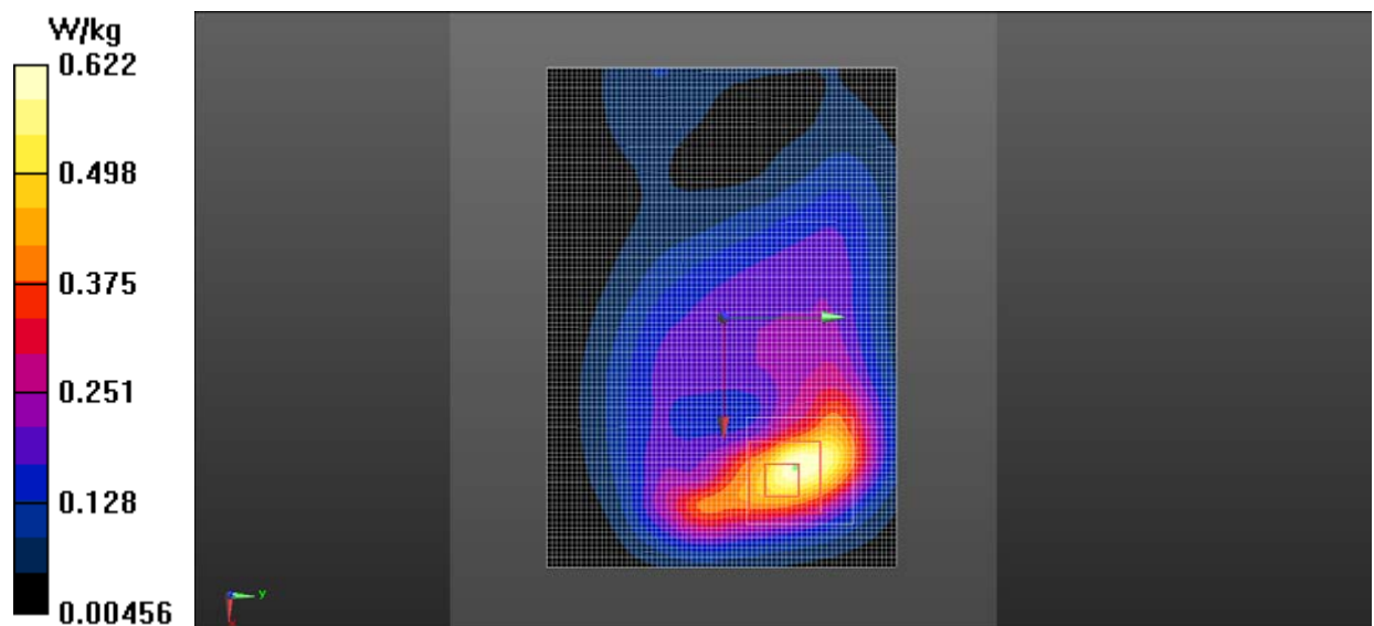
Fig.8 WCDMA1900 CH9538
