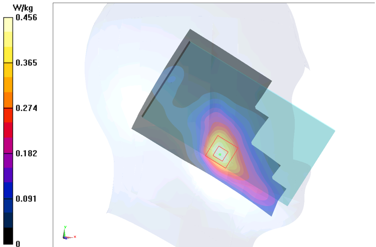
Fig.13 LTE Band7 CH21350
