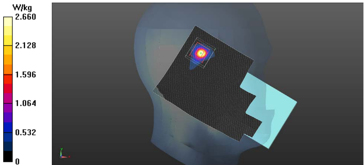
Fig.17 5GHz CH52
