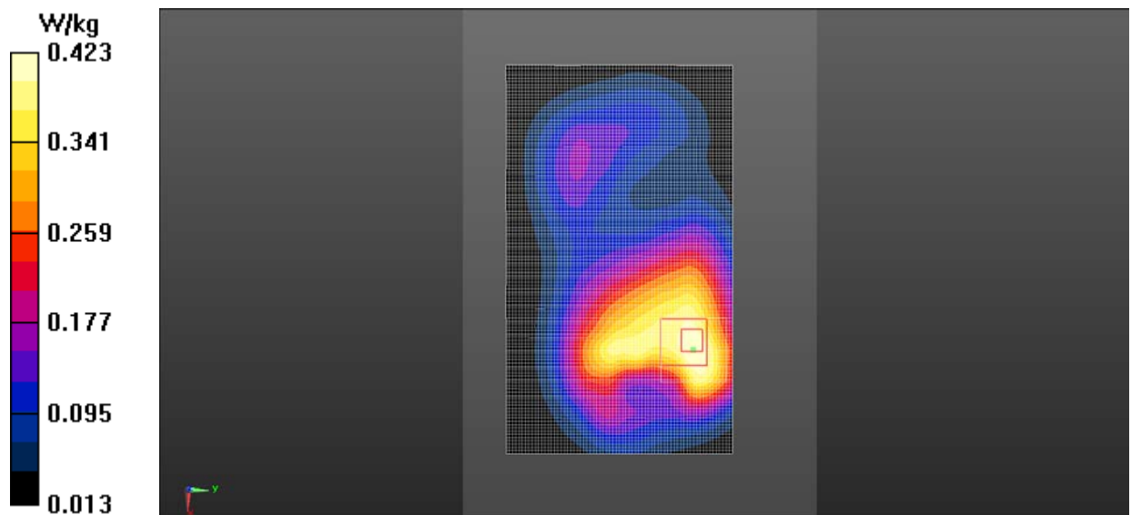
Fig.12 LTE Band4 CH20050
