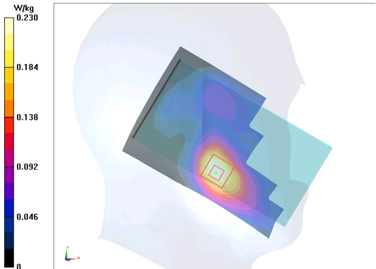
Fig.11 LTE Band4 CH20050
