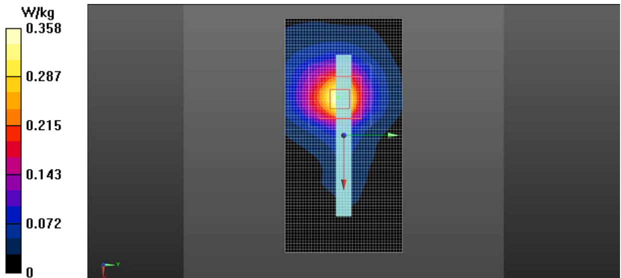
Fig.18 5GHz CH52
