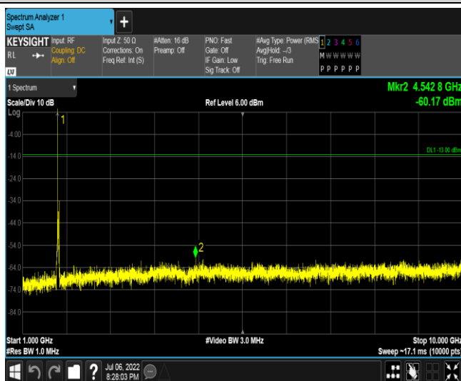
Band66-20MHz-QPSK-132072-1RB#0-Range3:1000~10000MHz
