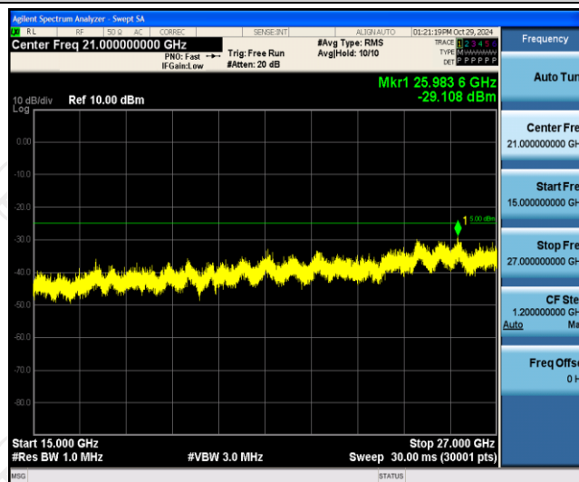
Band7-10MHz-QPSK-20800-1RB#0-Range3:15000~27000MHz
