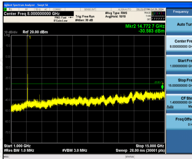
Band7-10MHz-QPSK-20800-1RB#0-Range2:1000~15000MHz
