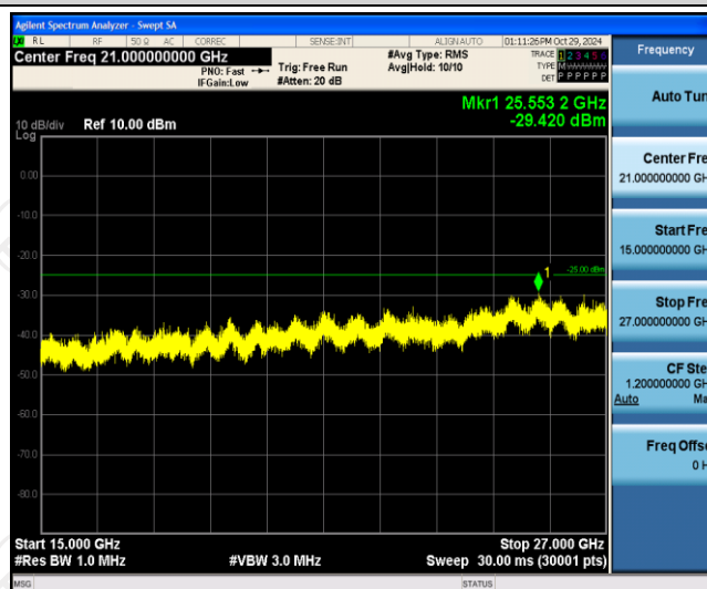
Band7-5MHz-QPSK-21425-1RB#0-Range3:15000~27000MHz
