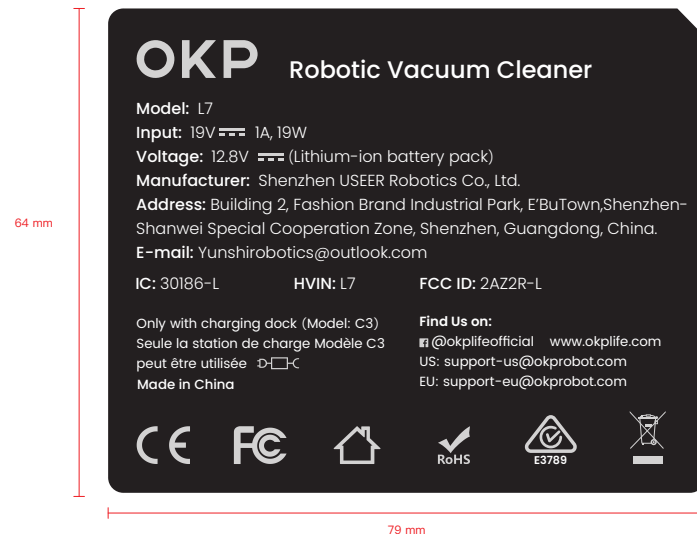
OKP品牌 L7 主机铭牌（欧美英澳）
