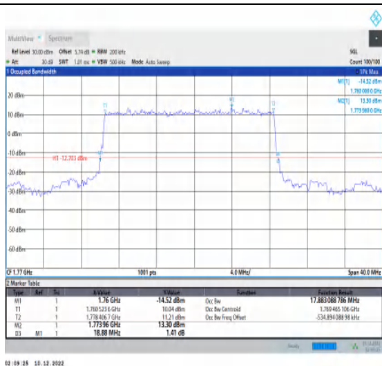
1-N66-15-20-H-2-DFT-PI2BPSK-Outer_Full-100@0-A Ant1-17.883-18.880-≤20-PASS
