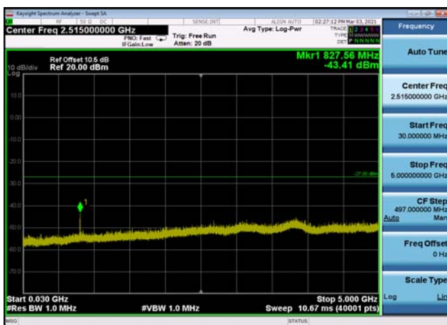
U-NII-1 ,Plot 2,30MHz~5000MHz-802.11a c(40MHz),5230MHz
