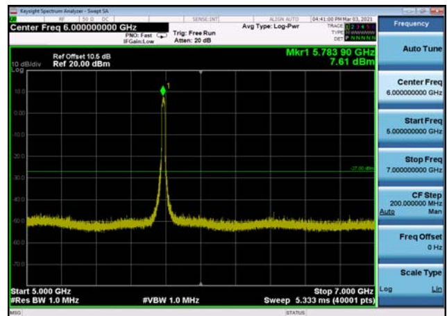
U-NII-3 ,Plot 3,5000MHz~7000MHz-802.1 1n(20MHz),5785MHz
