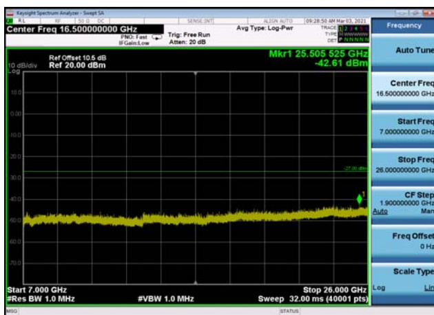
U-NII-1 ,Plot 4,7000MHz~26000MHz-802. 11a(20MHz),5220MHz
