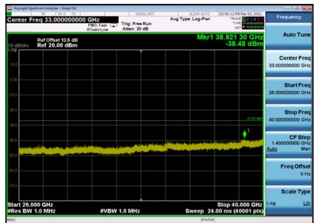
U-NII-1 ,Plot 2,26000MHz~40000MHz-802 .11a(20MHz),5240MHz
