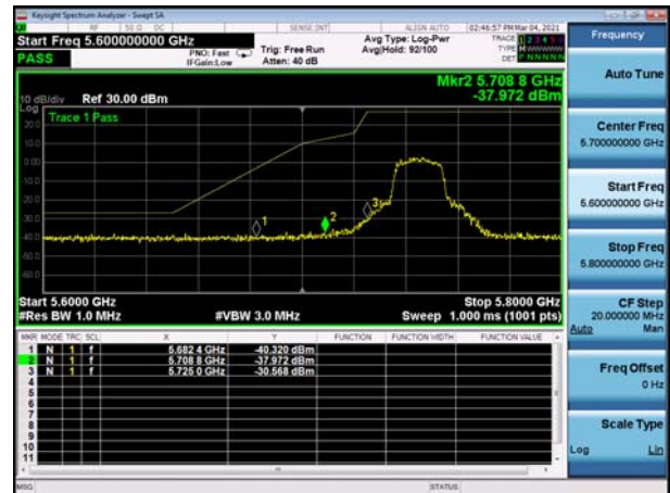
U-NII-3 ,Plot 1,Band Edge-802.11ac(20 MHz),5745MHz
