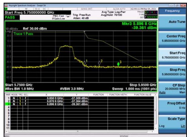
U-NII-3 ,Plot 1,Band Edge-802.11ac(20 MHz),5825MHz
