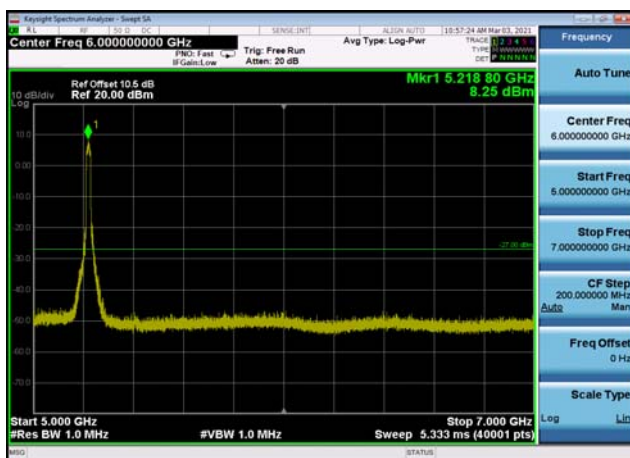
U-NII-1 ,Plot 3,5000MHz~7000MHz-802.1 1ac(20MHz),5220MHz
