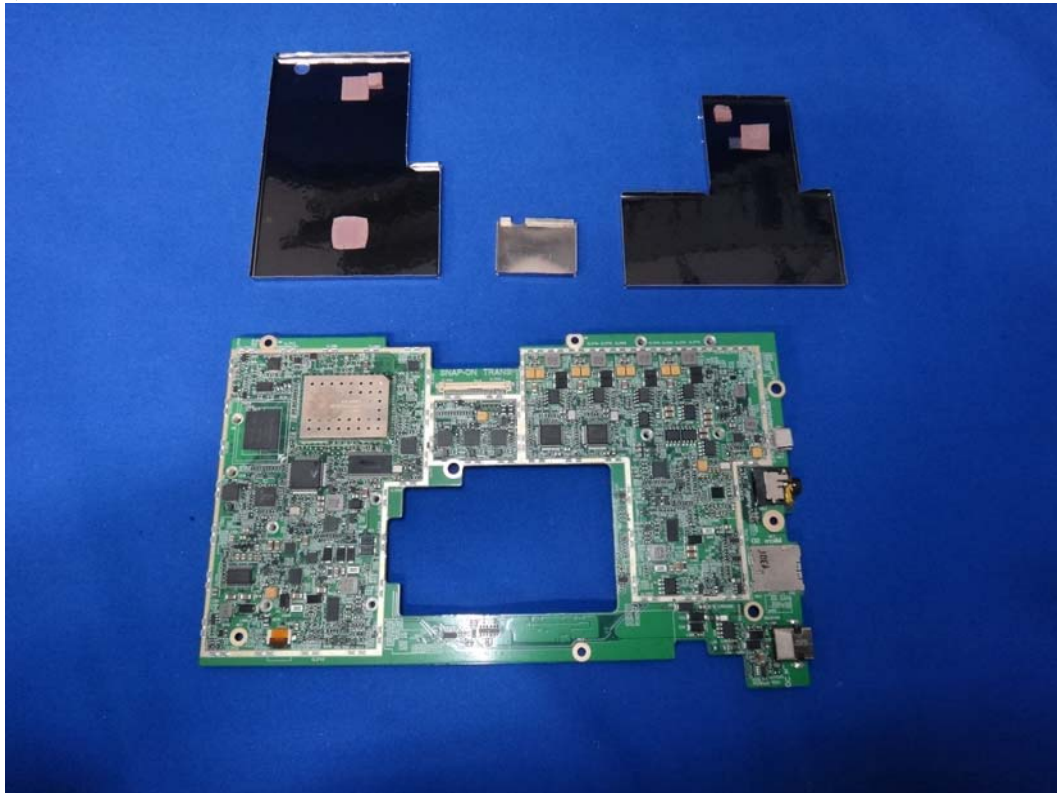
(36) EUT Photo
