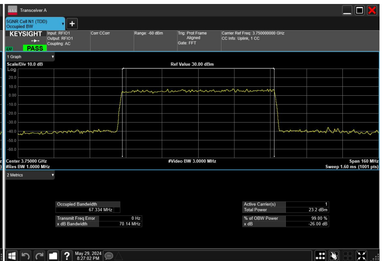
70MHz_30kHz_3750MHz_CP-OFDM QPSK_RB189@0
