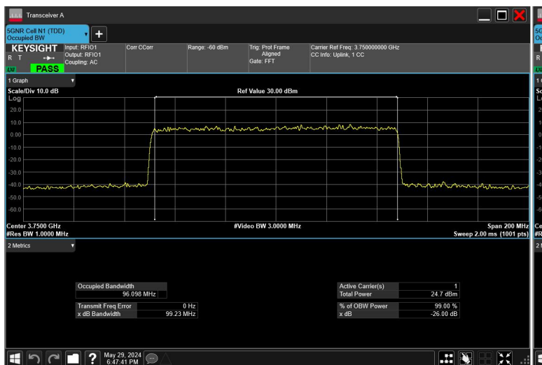
100MHz_30kHz_3750MHz_DFT-s-OFDM QPSK_RB270@0
