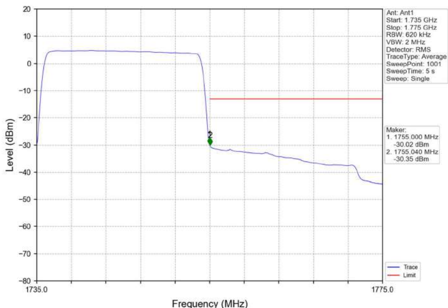
Band4_20MHz_QPSK_HCH_1745MHz_RB_100_0_NTNV
