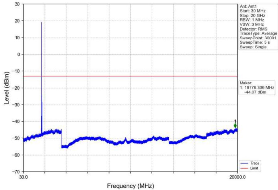
Band4_20MHz_QPSK_HCH_1745MHz_RB_1_0_NTNV
