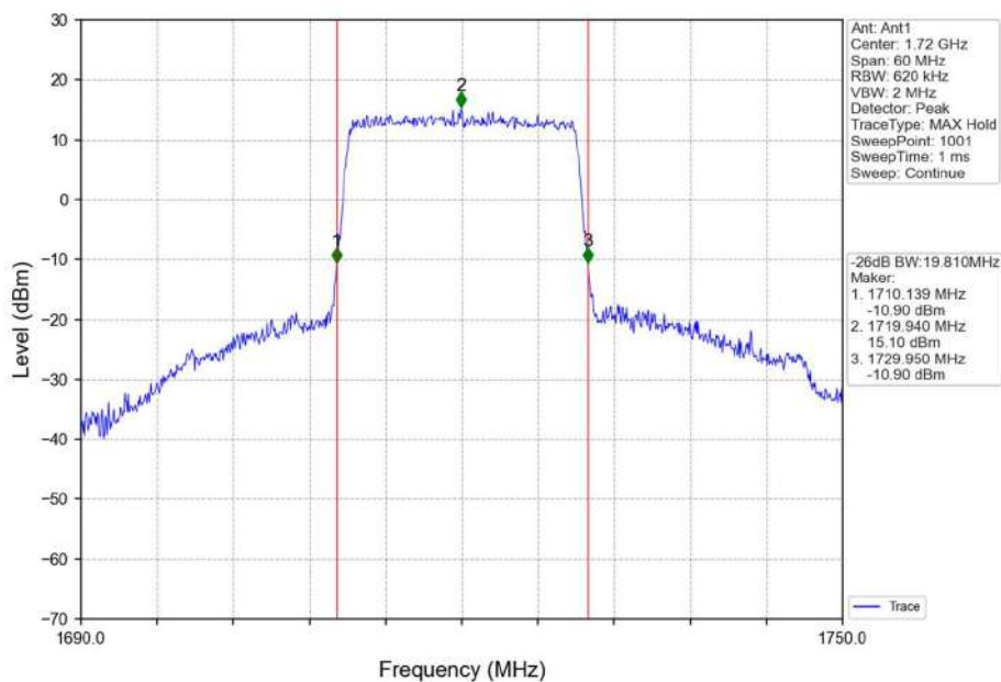
Band4_20MHz_QPSK_LCH_1720MHz_RB_100_0_NTNV
