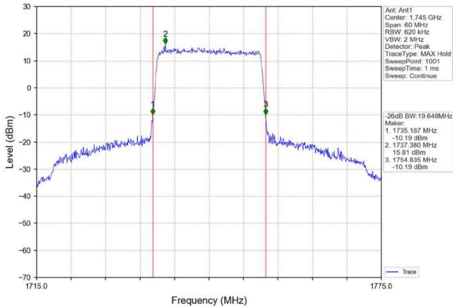
Band4_20MHz_QPSK_HCH_1745MHz_RB_100_0_NTNV
