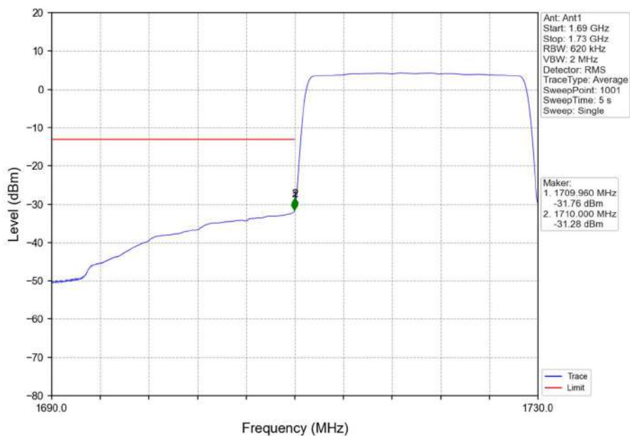
Band4_20MHz_QPSK_LCH_1720MHz_RB_100_0_NTNV
