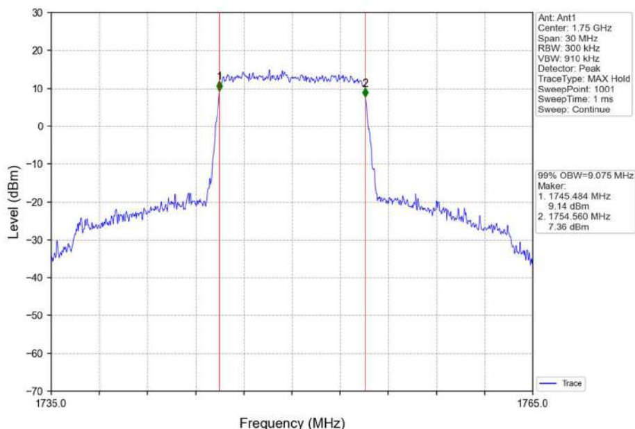
Band4_10MHz_QPSK_HCH_1750MHz_RB_50_0_NTNV
