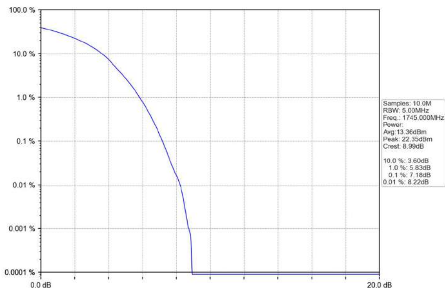
Band4_20MHz_QPSK_HCH_1745MHz_RB_100_0_NTNV
