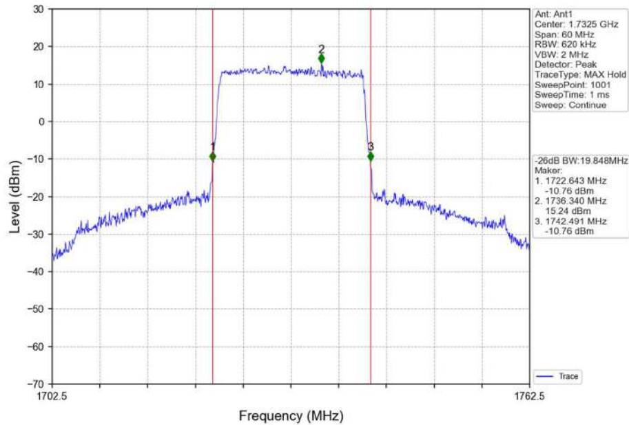
Band4_20MHz_QPSK_MCH_1732.5MHz_RB_100_0_NTNV
