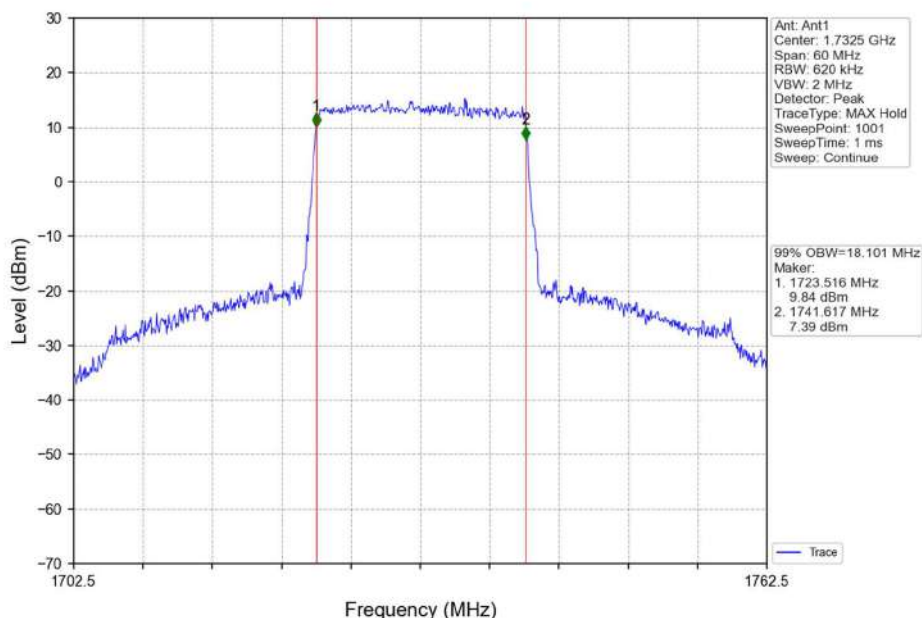
Band4_20MHz_QPSK_MCH_1732.5MHz_RB_100_0_NTNV
