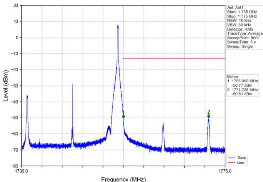
Band4_20MHz_QPSK_HCH_1745MHz_RB_1_99_NTNV
