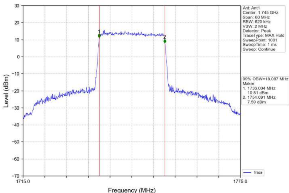
Band4_20MHz_QPSK_HCH_1745MHz_RB_100_0_NTNV
