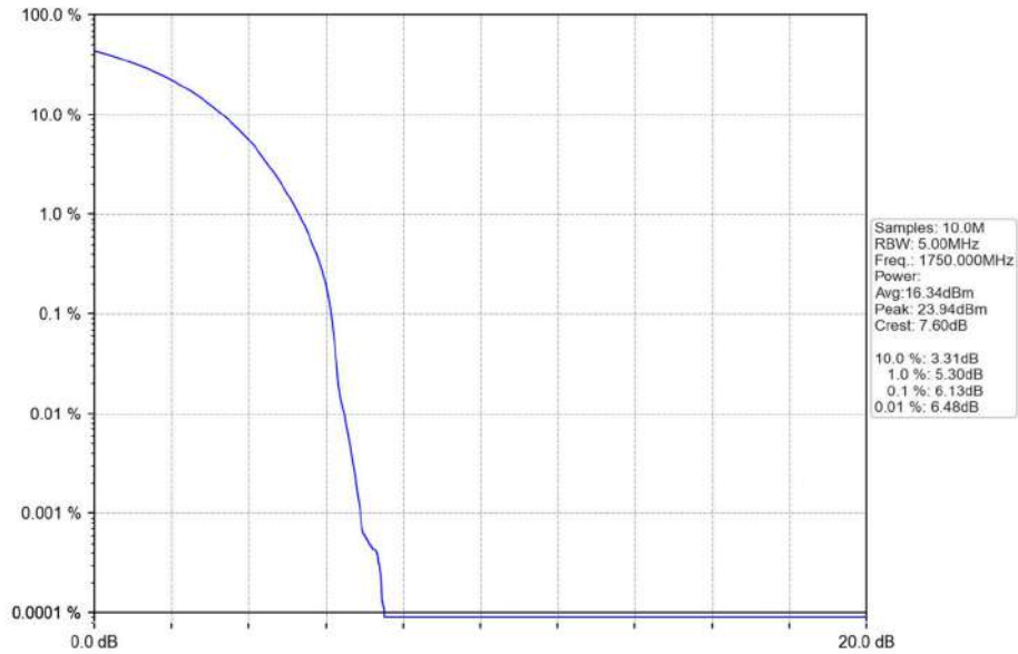
Band4_10MHz_QPSK_HCH_1750MHz_RB_50_0_NTNV
