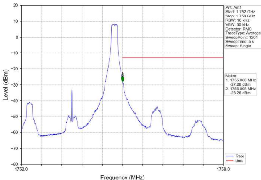
Band4_3MHz_QPSK_HCH_1753.5MHz_RB_1_14_NTNV
