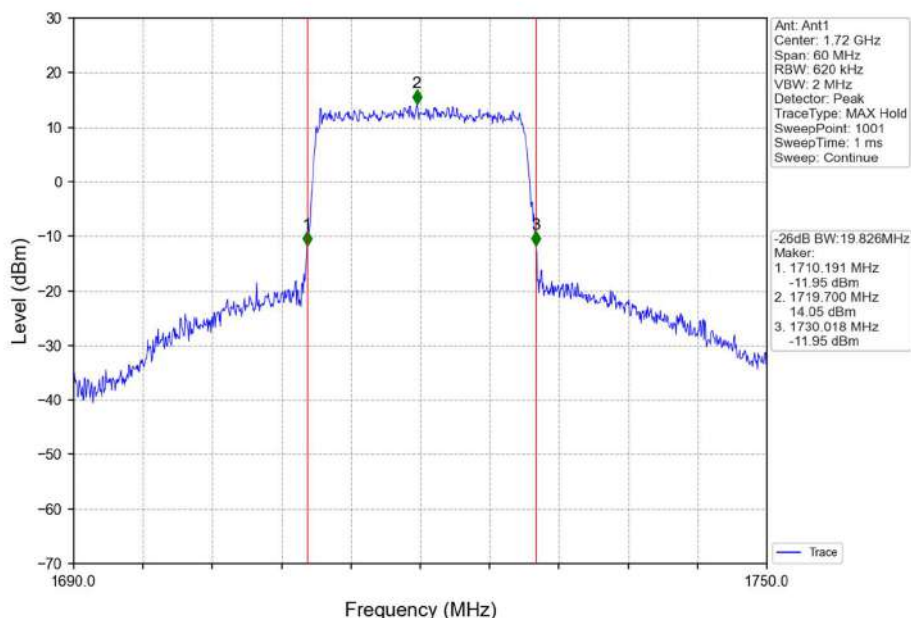
Band4_20MHz_16QAM_LCH_1720MHz_RB_100_0_NTNV
