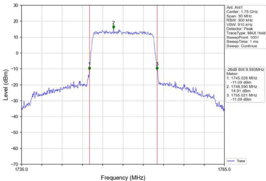
Band4_10MHz_QPSK_HCH_1750MHz_RB_50_0_NTNV
