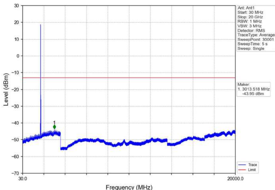
Band4_20MHz_QPSK_MCH_1732.5MHz_RB_1_0_NTNV
