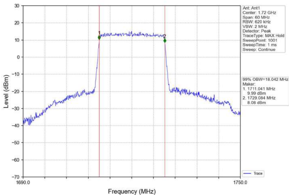
Band4_20MHz_QPSK_LCH_1720MHz_RB_100_0_NTNV
