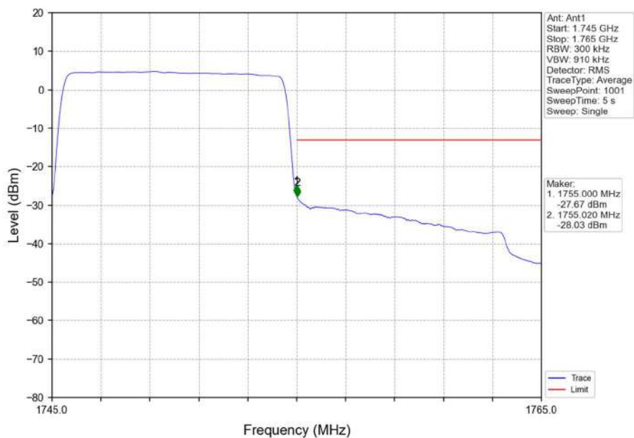
Band4_10MHz_QPSK_HCH_1750MHz_RB_50_0_NTNV
