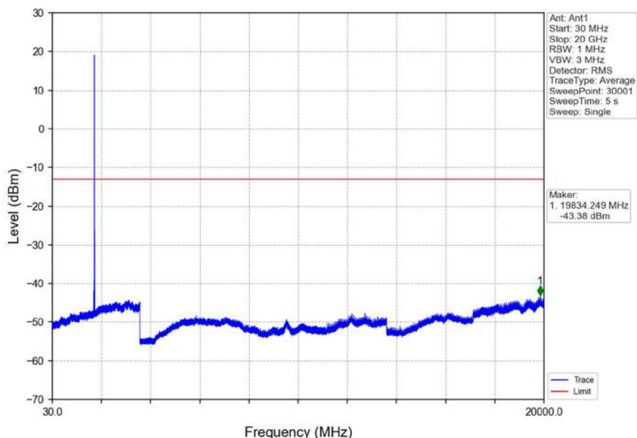
Band4_10MHz_QPSK_HCH_1750MHz_RB_1_0_NTNV
