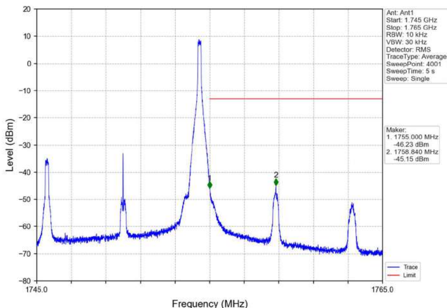
Band4_10MHz_QPSK_HCH_1750MHz_RB_1_49_NTNV
