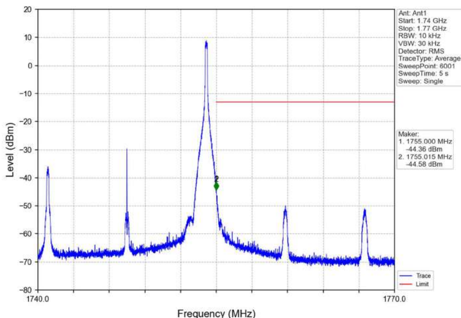
Band4_15MHz_QPSK_HCH_1747.5MHz_RB_1_74_NTNV
