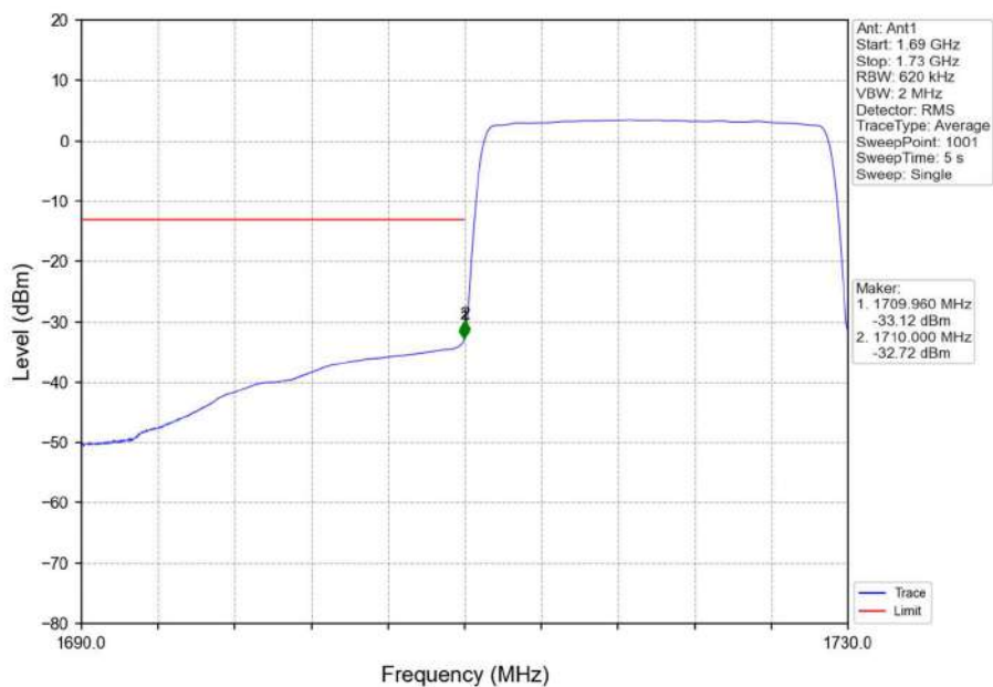
Band4_20MHz_16QAM_LCH_1720MHz_RB_100_0_NTNV
