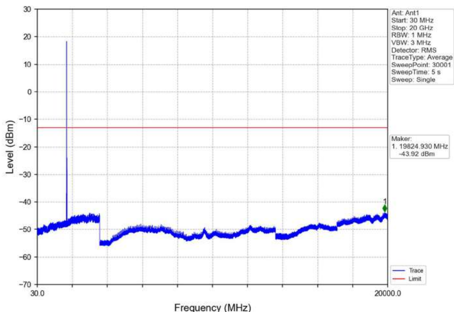
Band4_15MHz_QPSK_LCH_1717.5MHz_RB_1_0_NTNV
